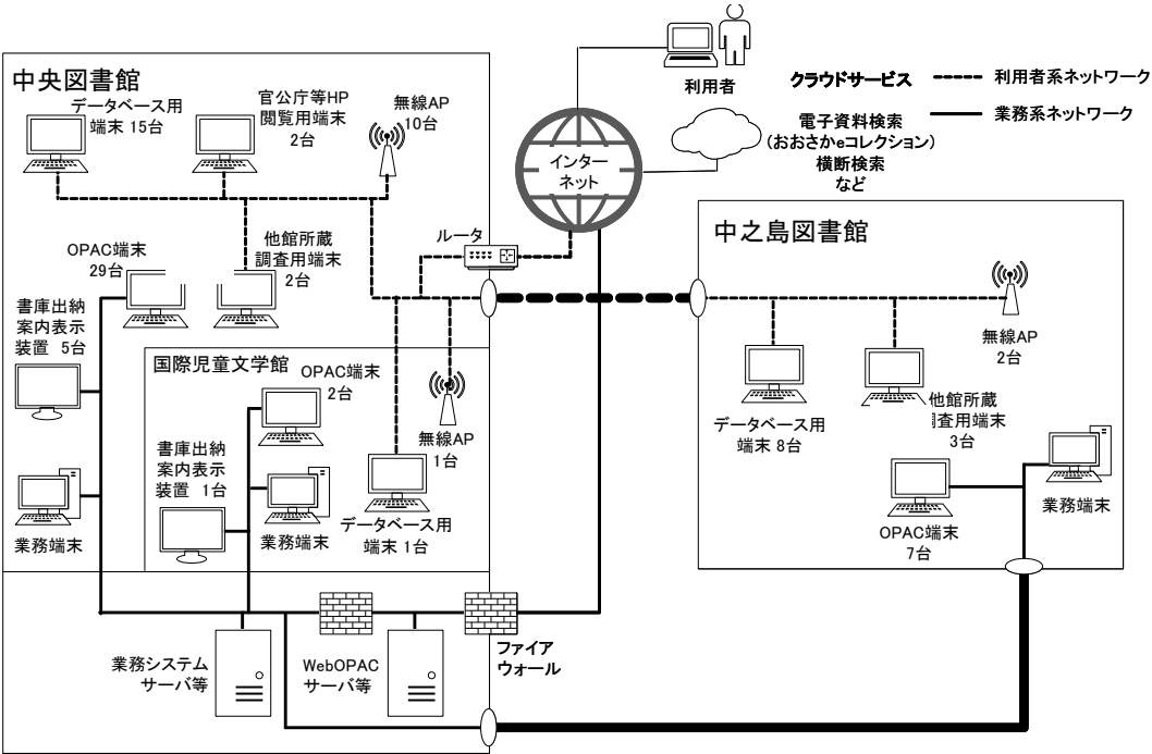
≪大阪府立図書館情報システム構成図≫ 令和4年4月1日現在
