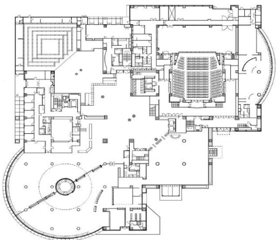
1 階平面図
