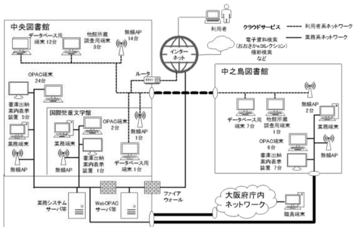
《大阪府立図書館情報システム構成図》
