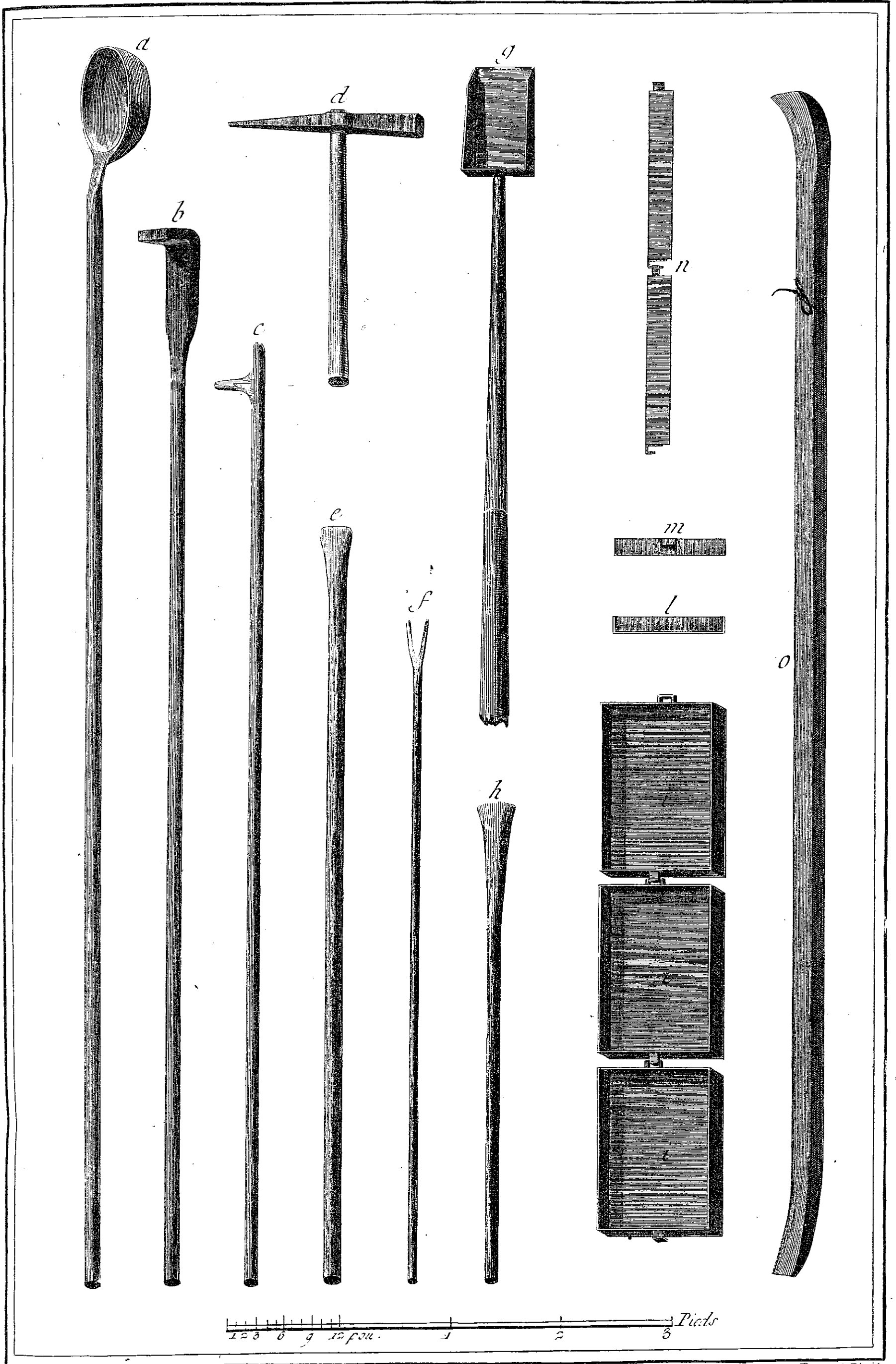
Verrerie en bois, Différens Outils employés dans les petites Ferreries à pivotelle.
