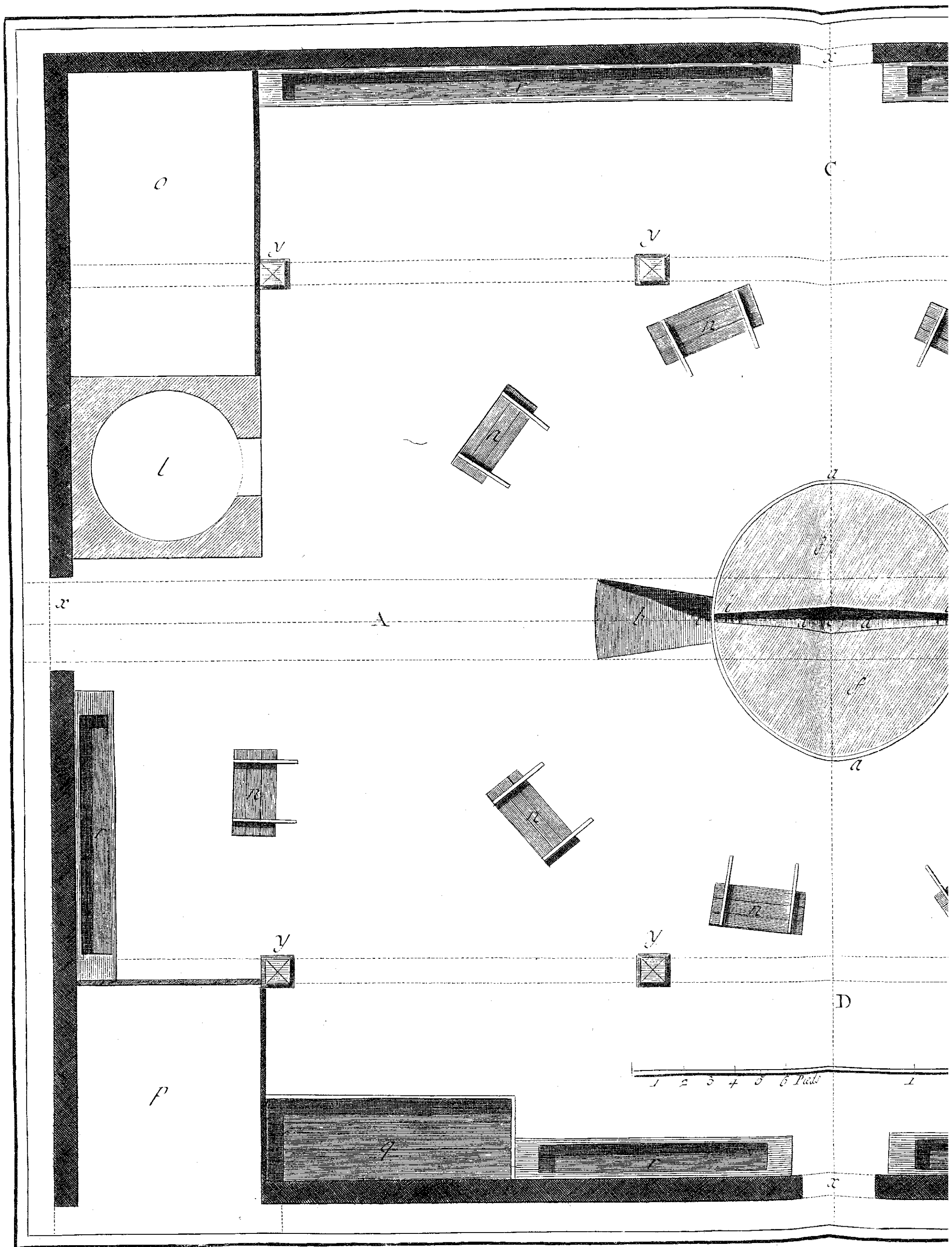
Verrerie en bois, Plan Géométral d'une Halle de petite Verrerie à po
