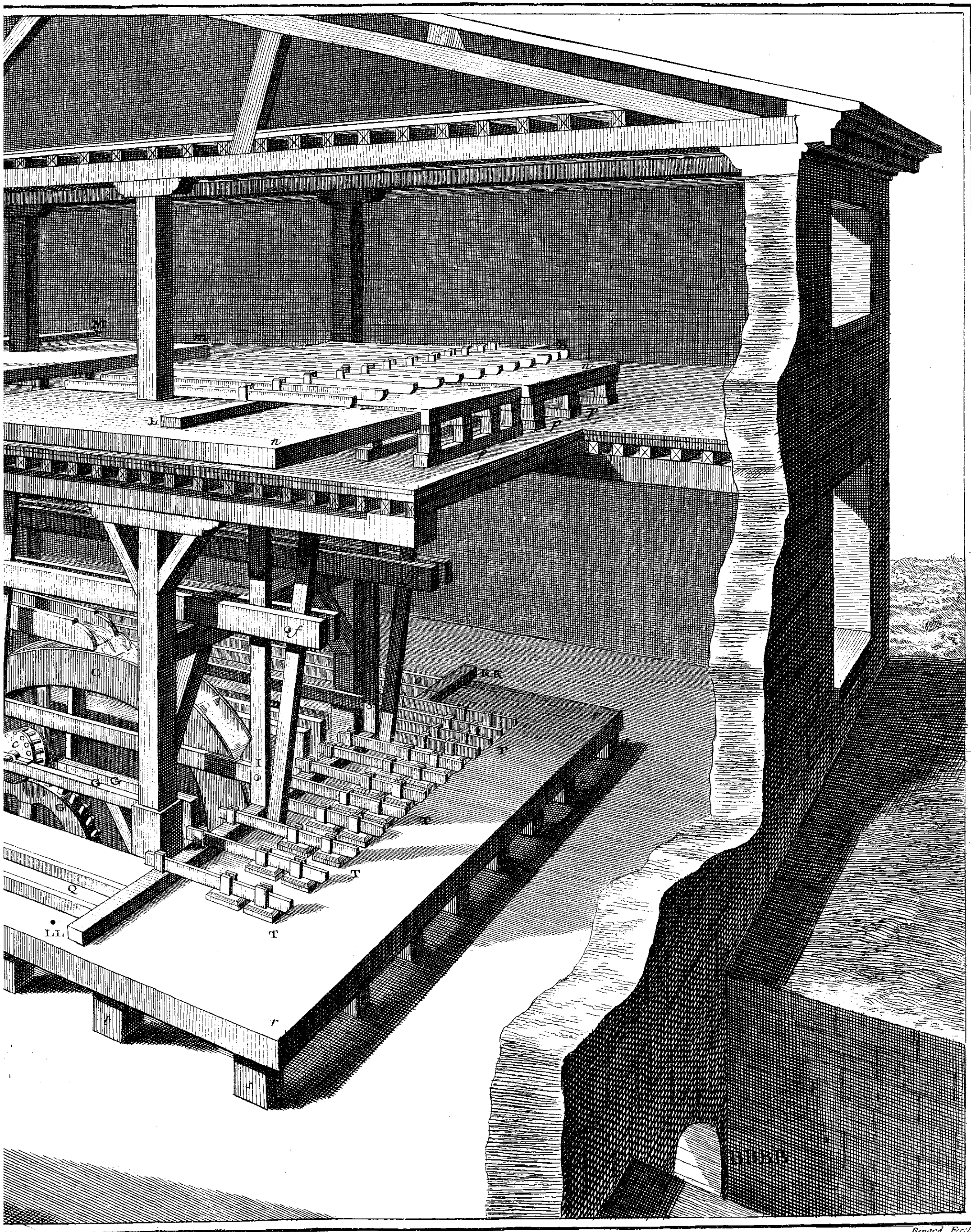
de la Machine à polir les Glaces, Etablie à S e Idelfonse.
