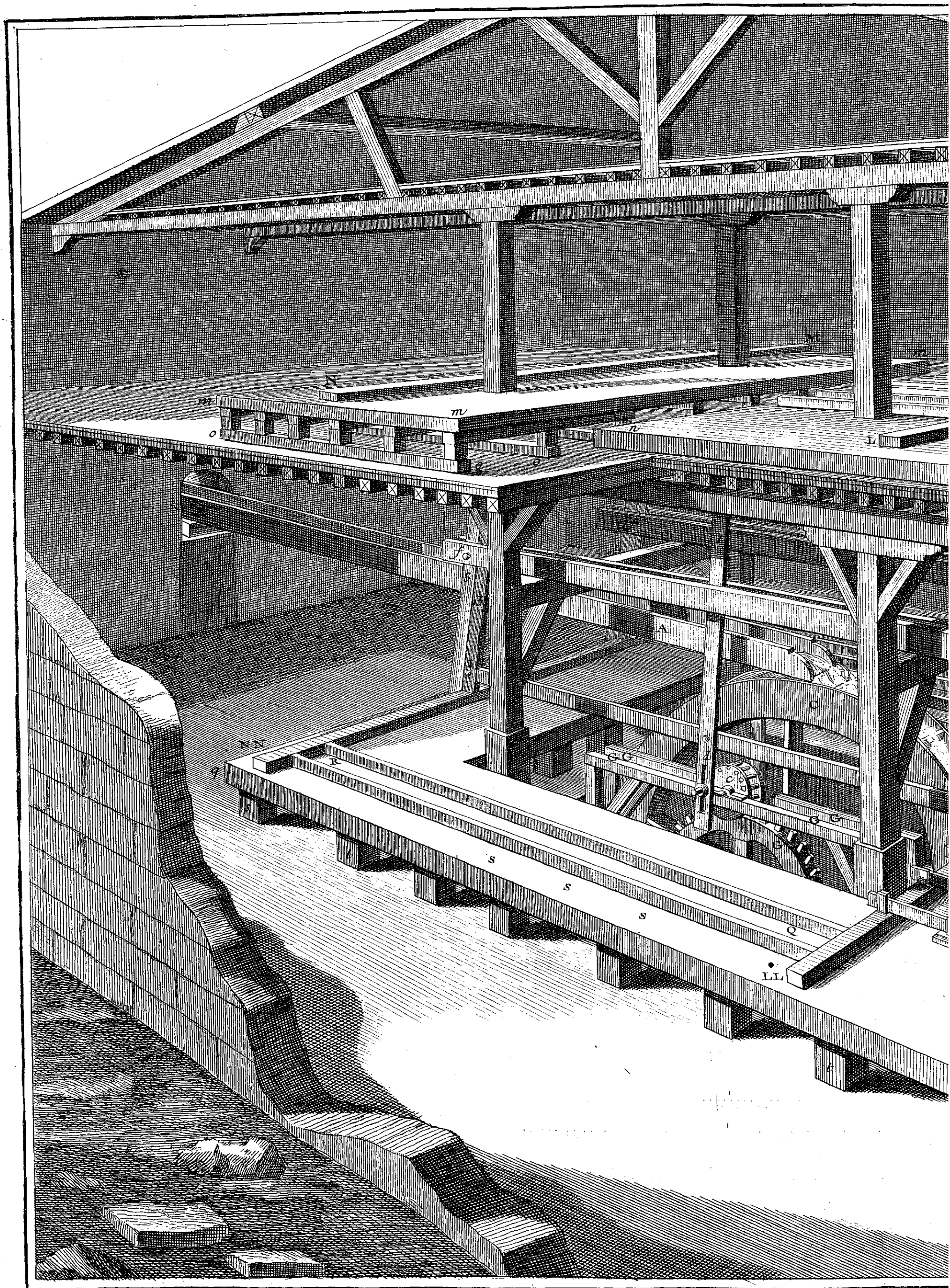
Glaces, Elevation perspective de la Machine à polir.
