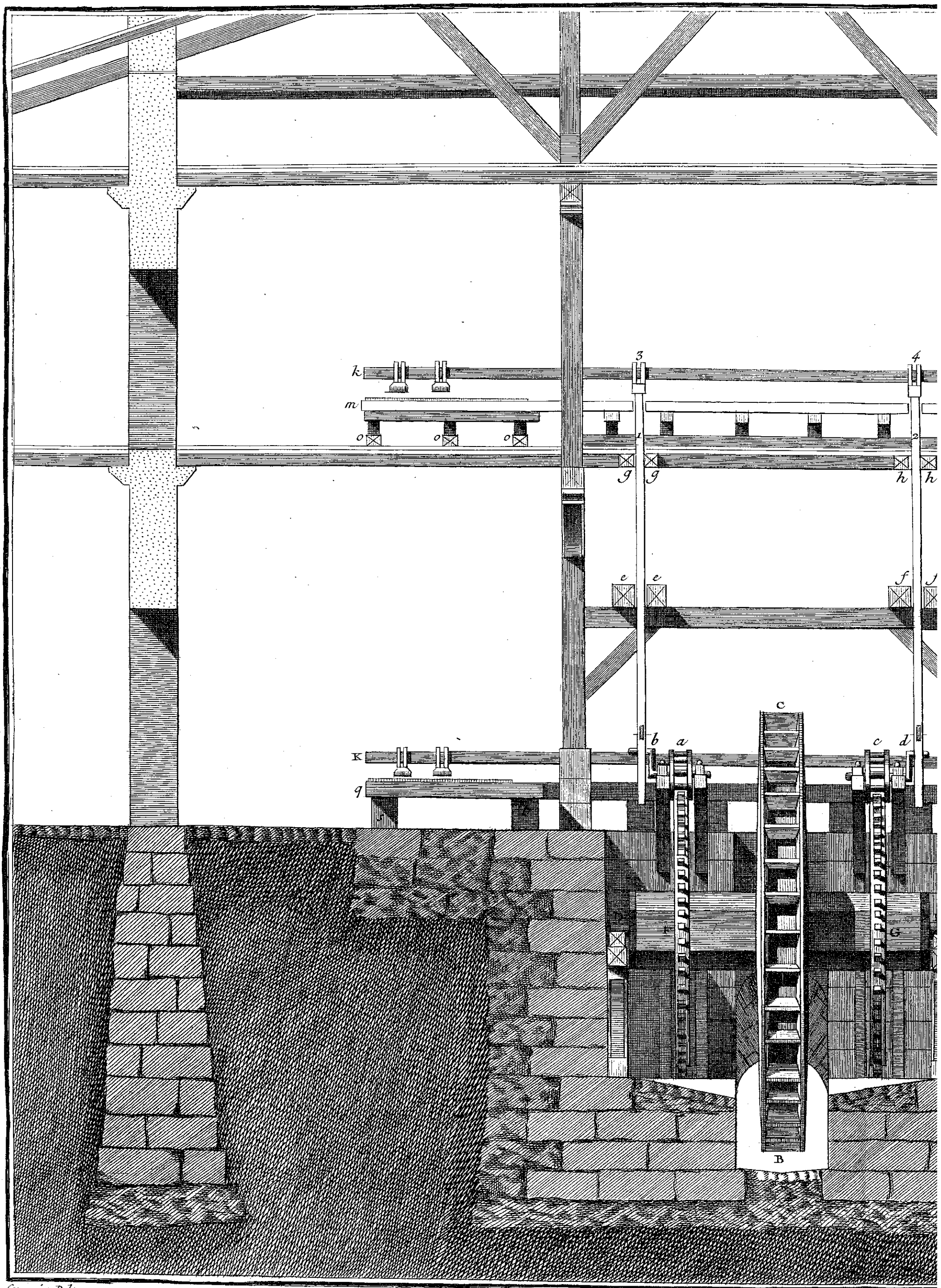
Glaces, Coupe et Elevation de la Machine à polir les Glaces.
