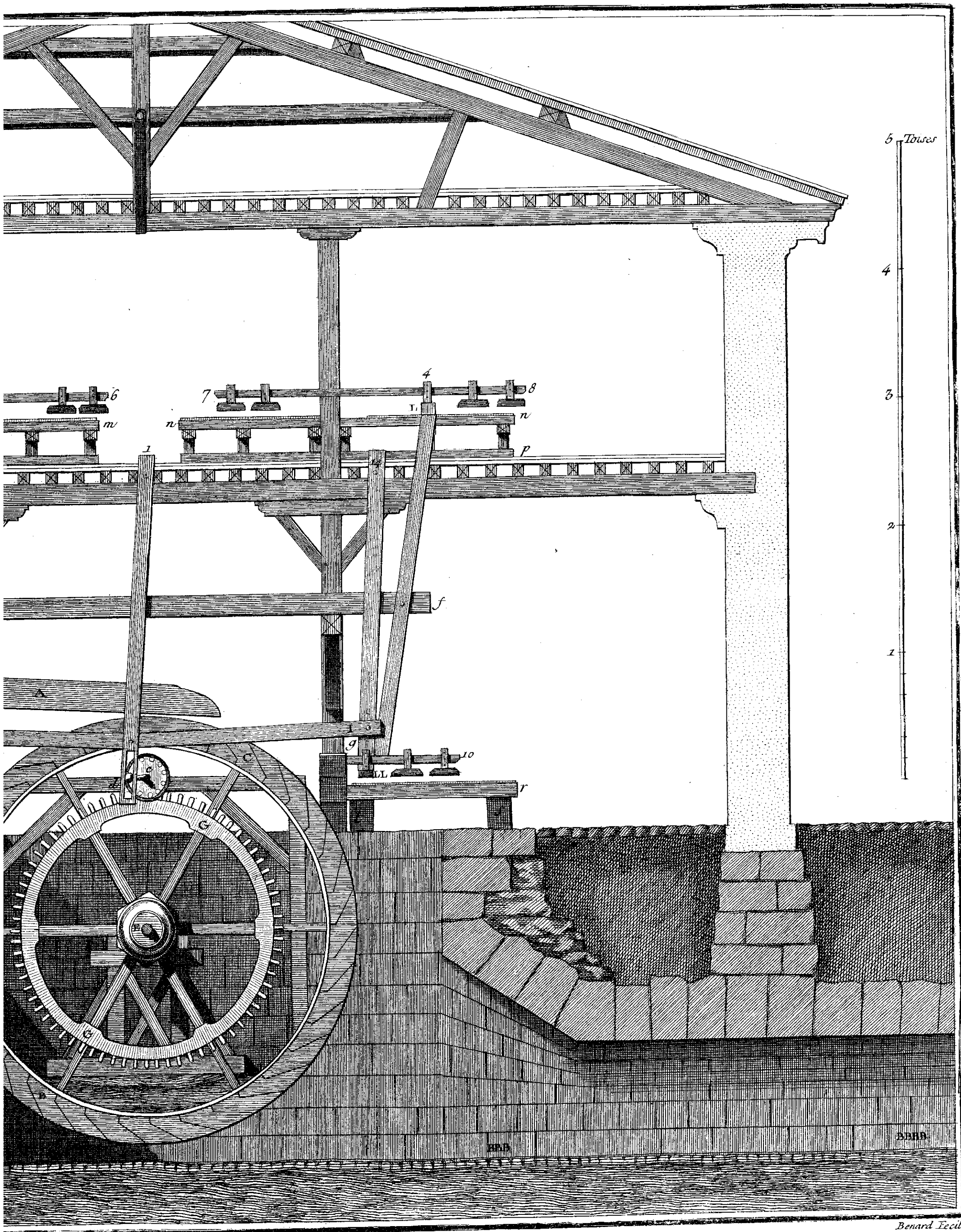
Machine à polir les Glaces prise selon la longueur du Courssier.
