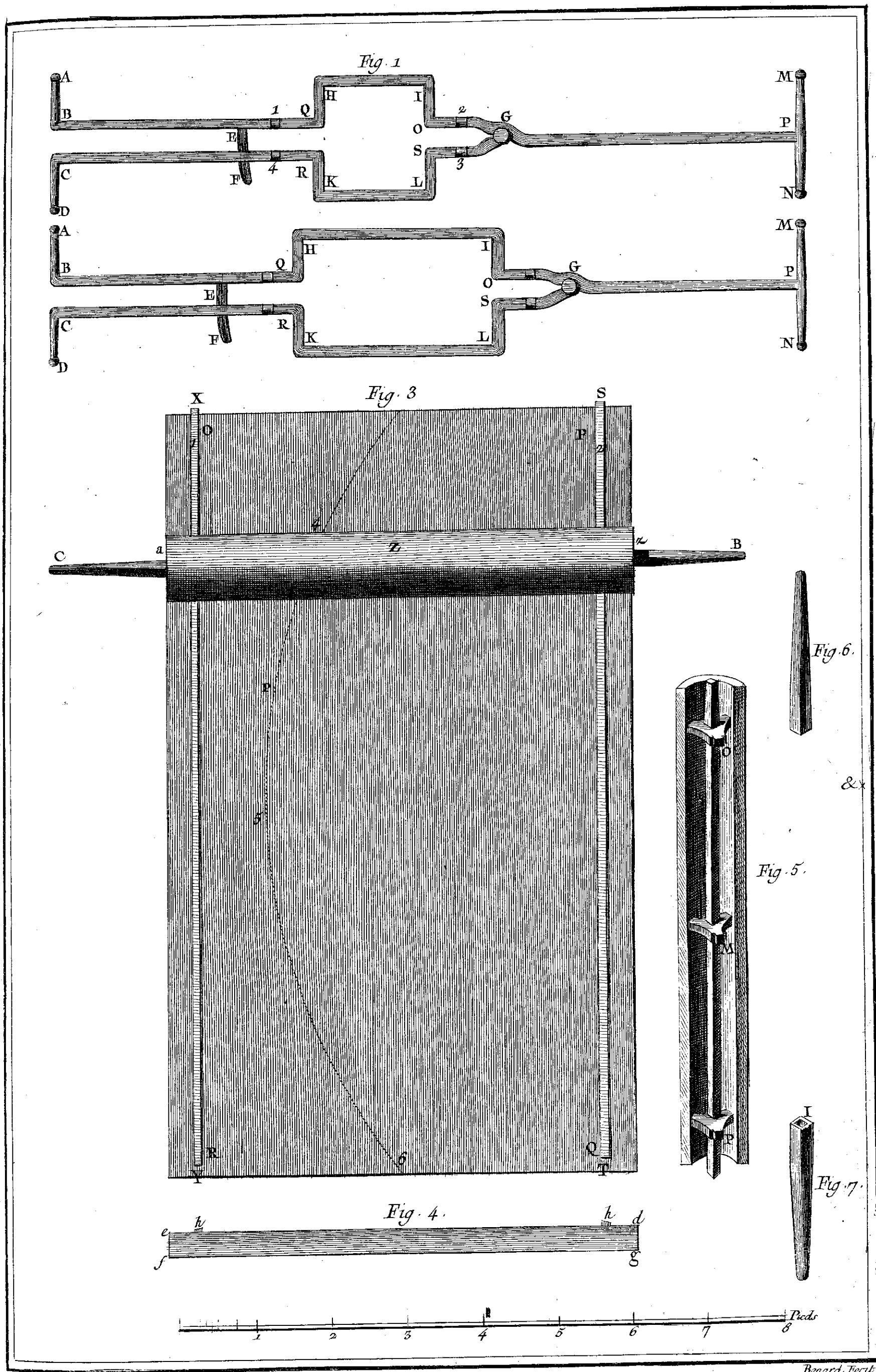
Glaces, Plan des Tenailles et de la Table.
