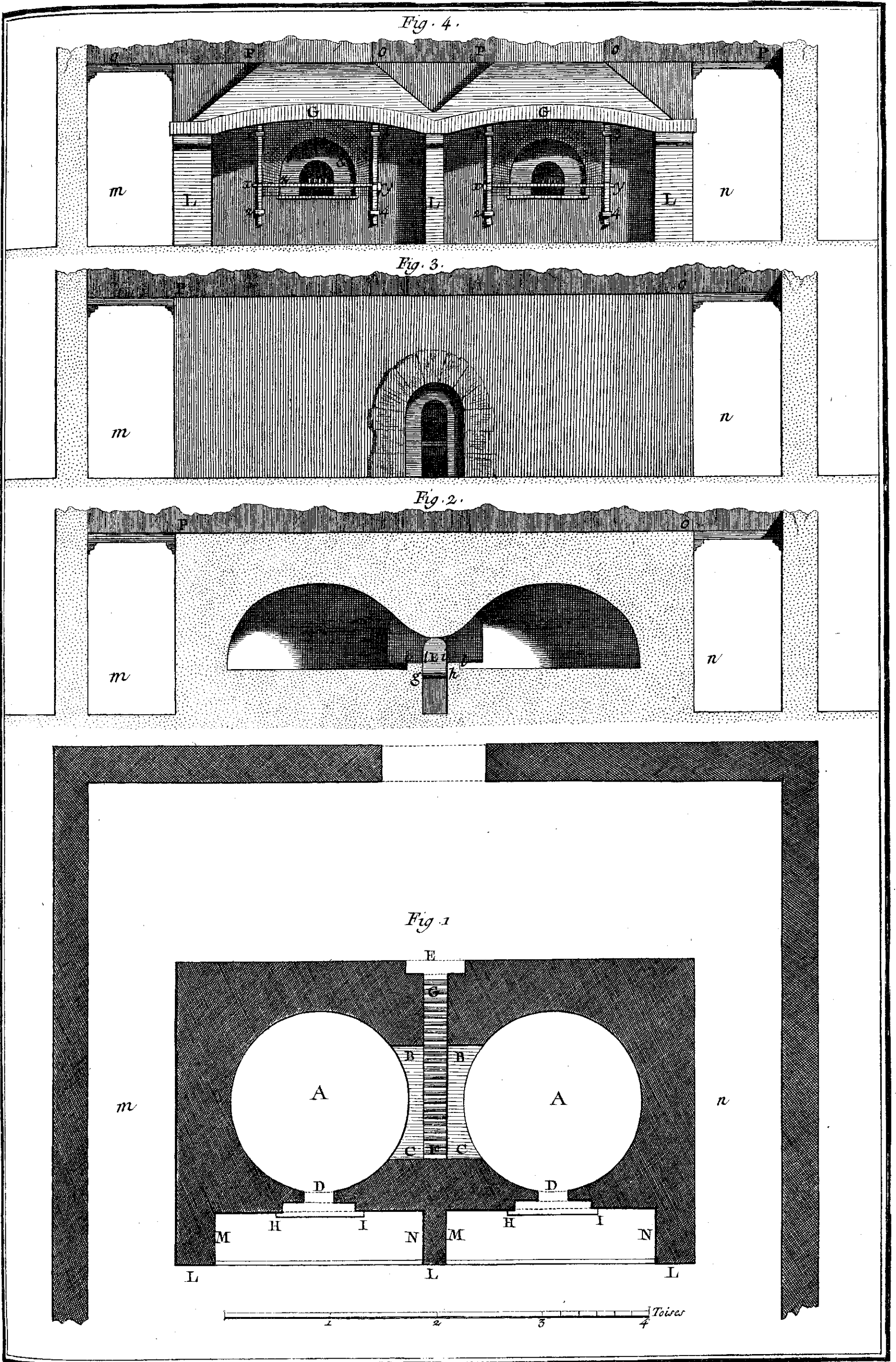
Glaces, Élévations, Coupe et Plan d'un Four à Fritte double.
