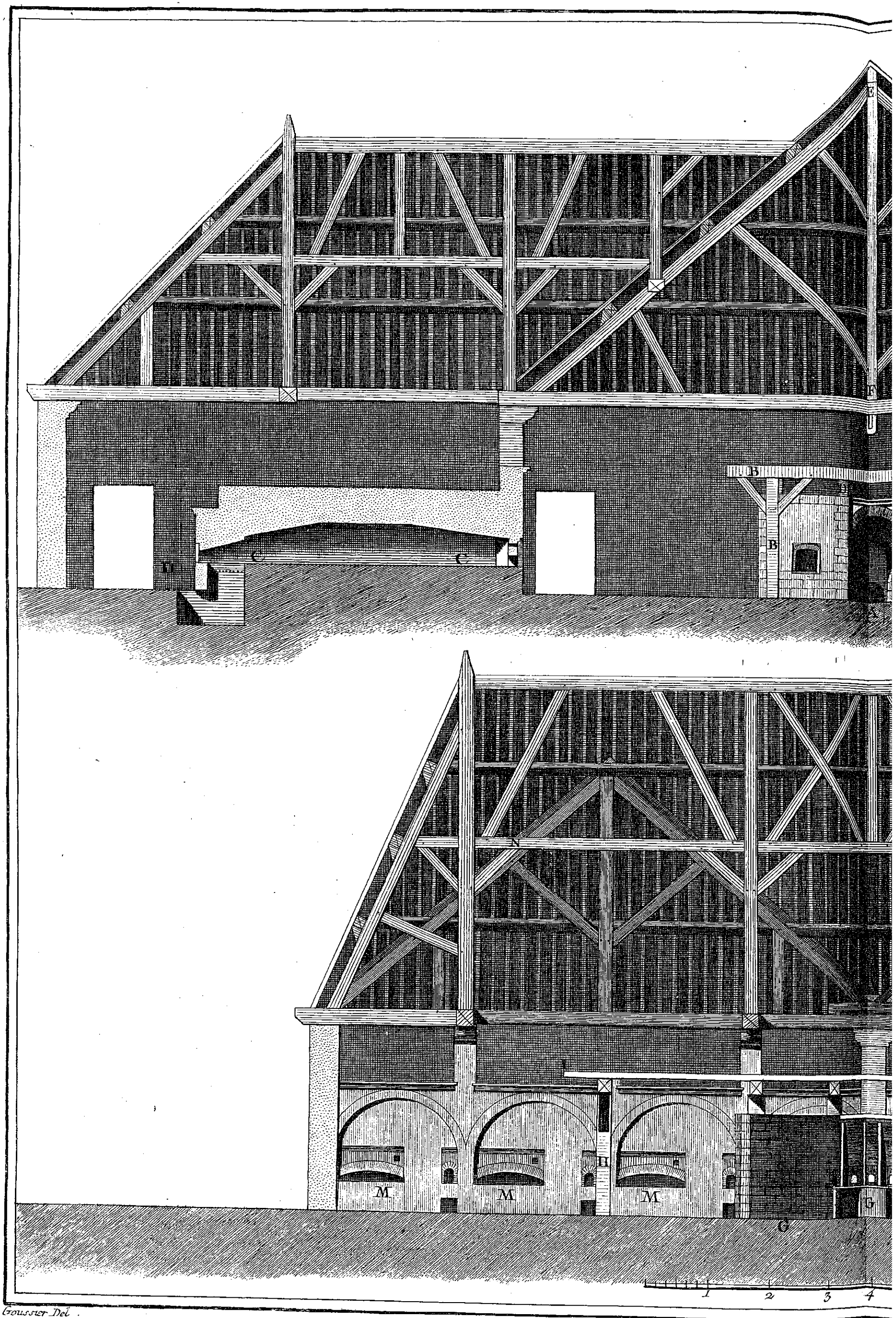
Glaces, coupes Longitudinales
