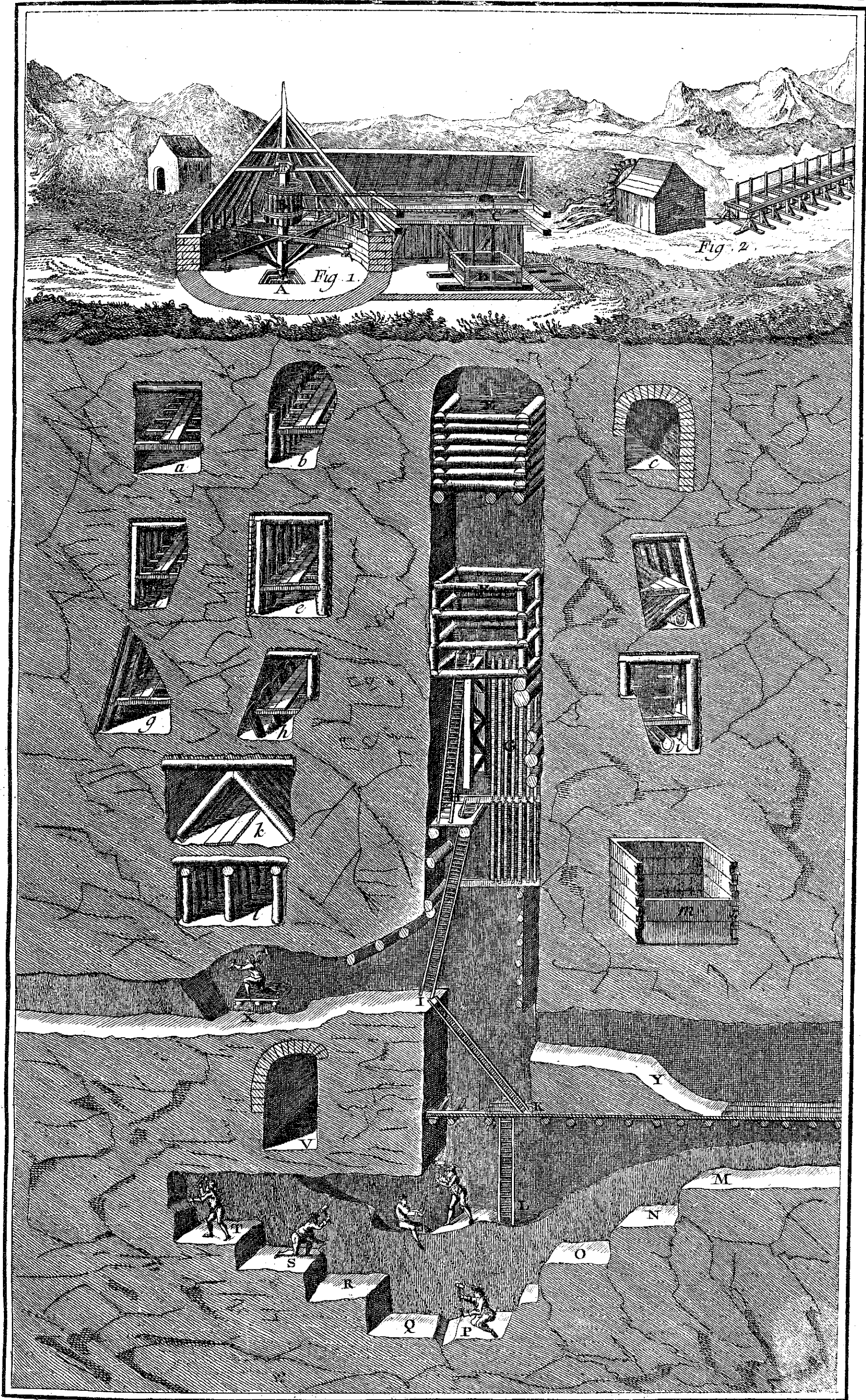
Minéralogie, coupe d'une Mine.
