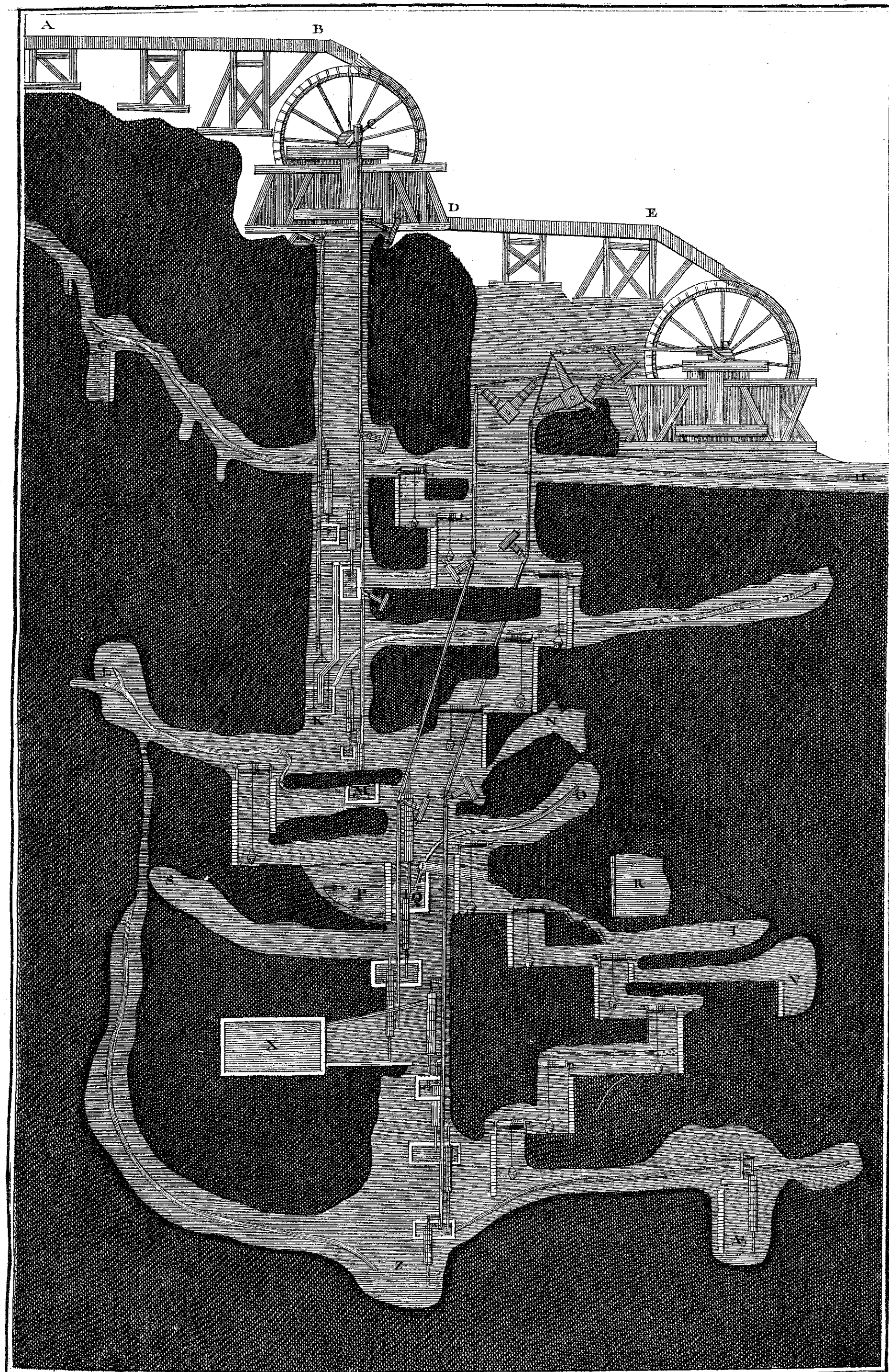
Minéralogie, Disposition des Machines servant aux Epuisements
