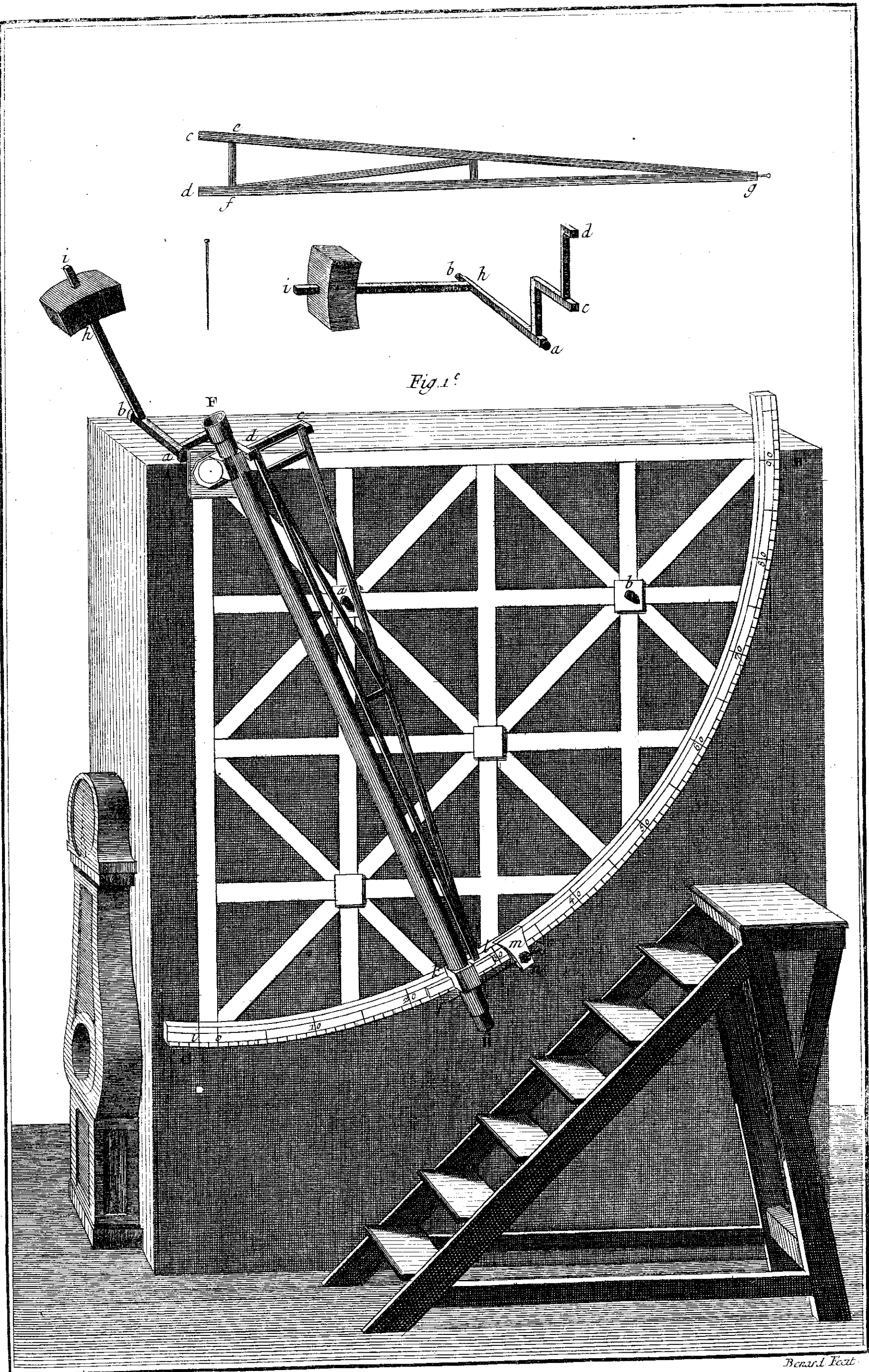
Astronomie Instrumens , Quart de cercle Mural en Perspective et développement du Contrepoid de la Lunette .
