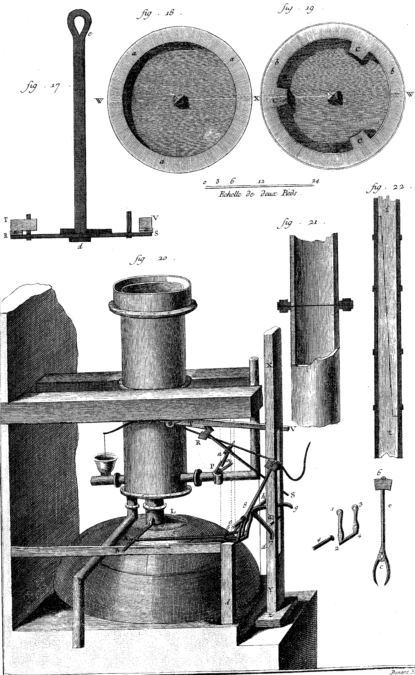
Hidraulique, Pompe à Feu Soudes et profils du Cilindre.
