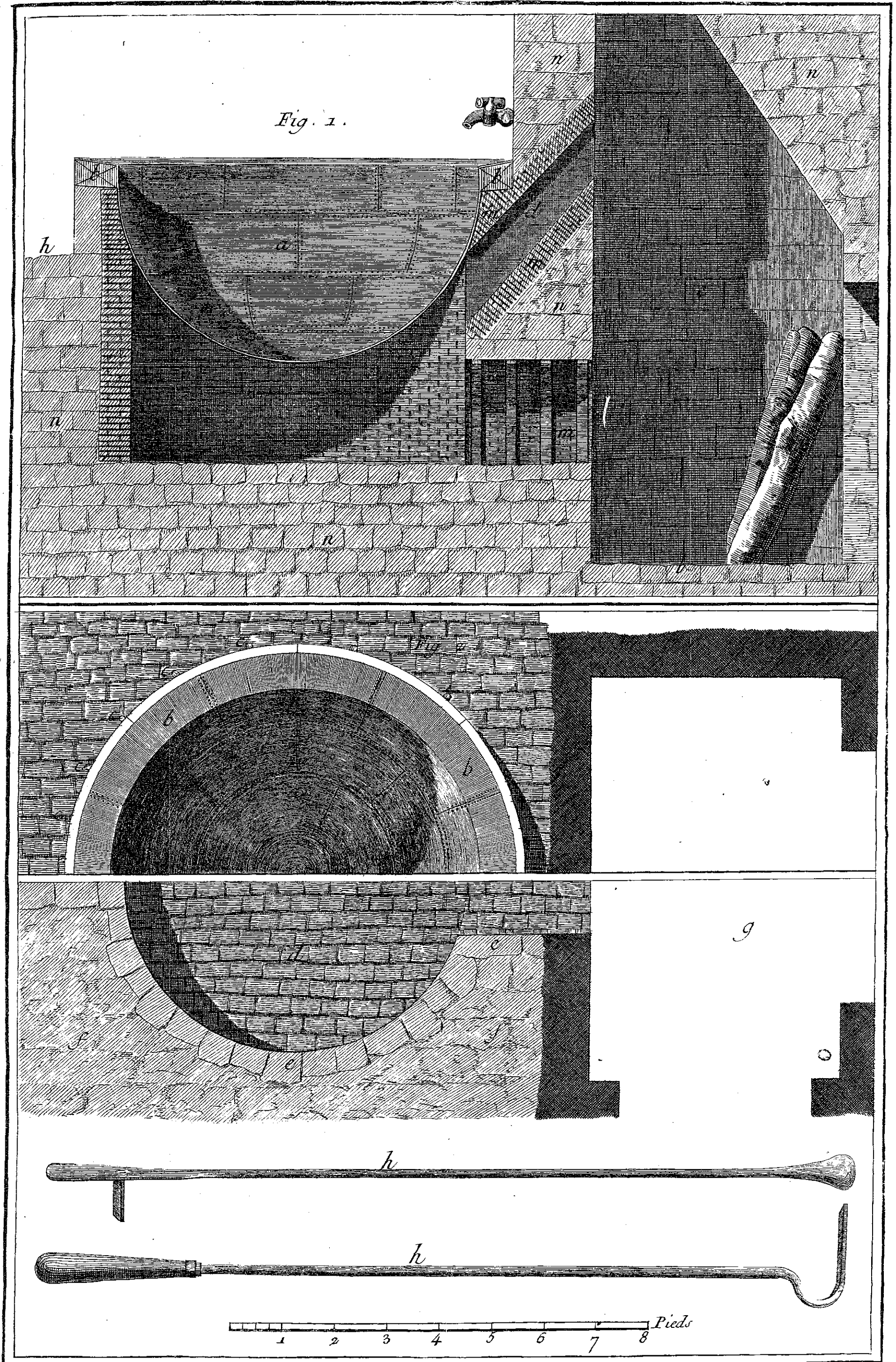
Teinture des Gobelins, Plans et Coupe d'un Fourneau, et Outils
