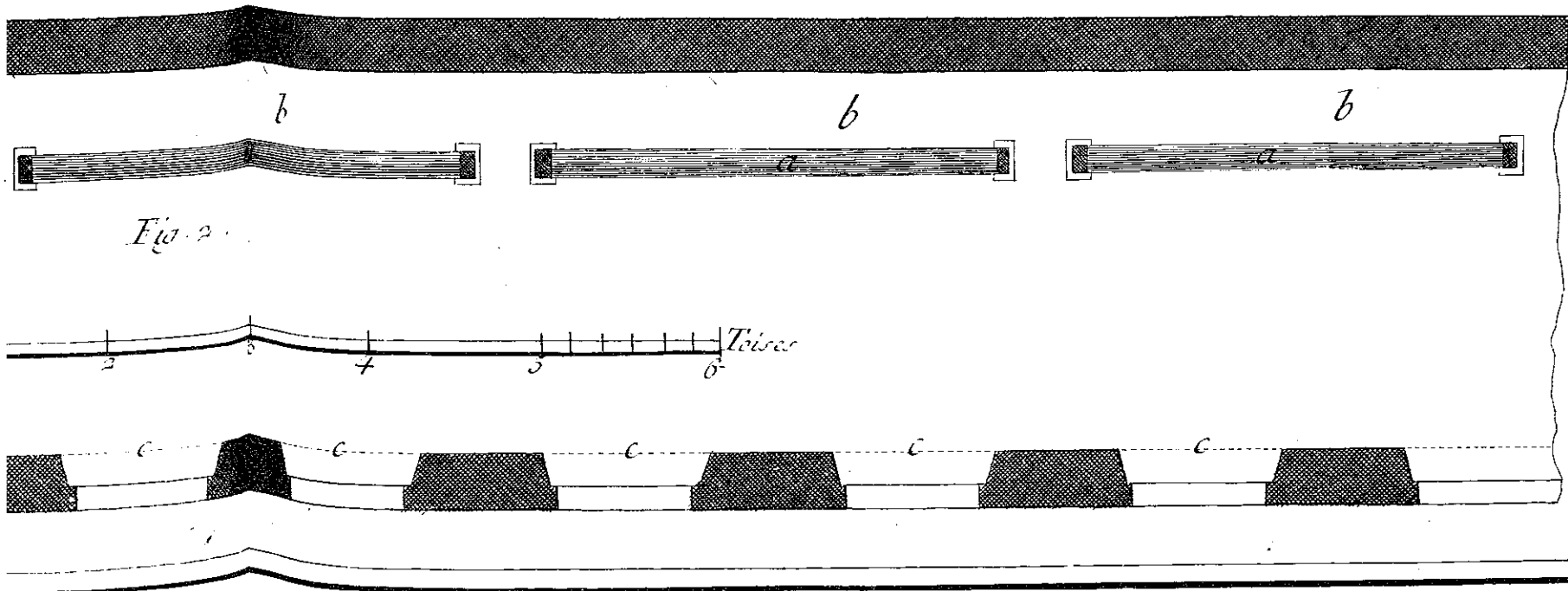
Gobelins, Plan et Perspective de l'Atelier, des Metiers, et différentes Opérations.
