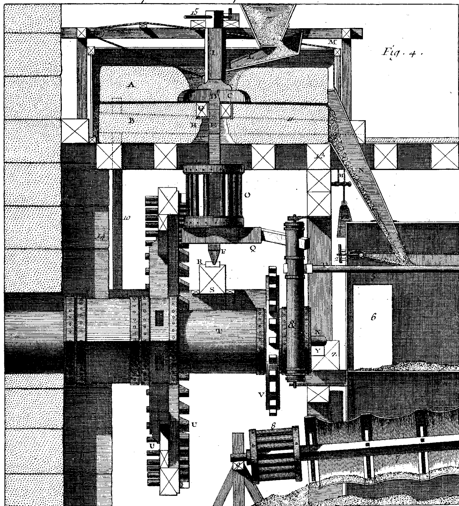
Principale Méchanique d'un Moulin.
