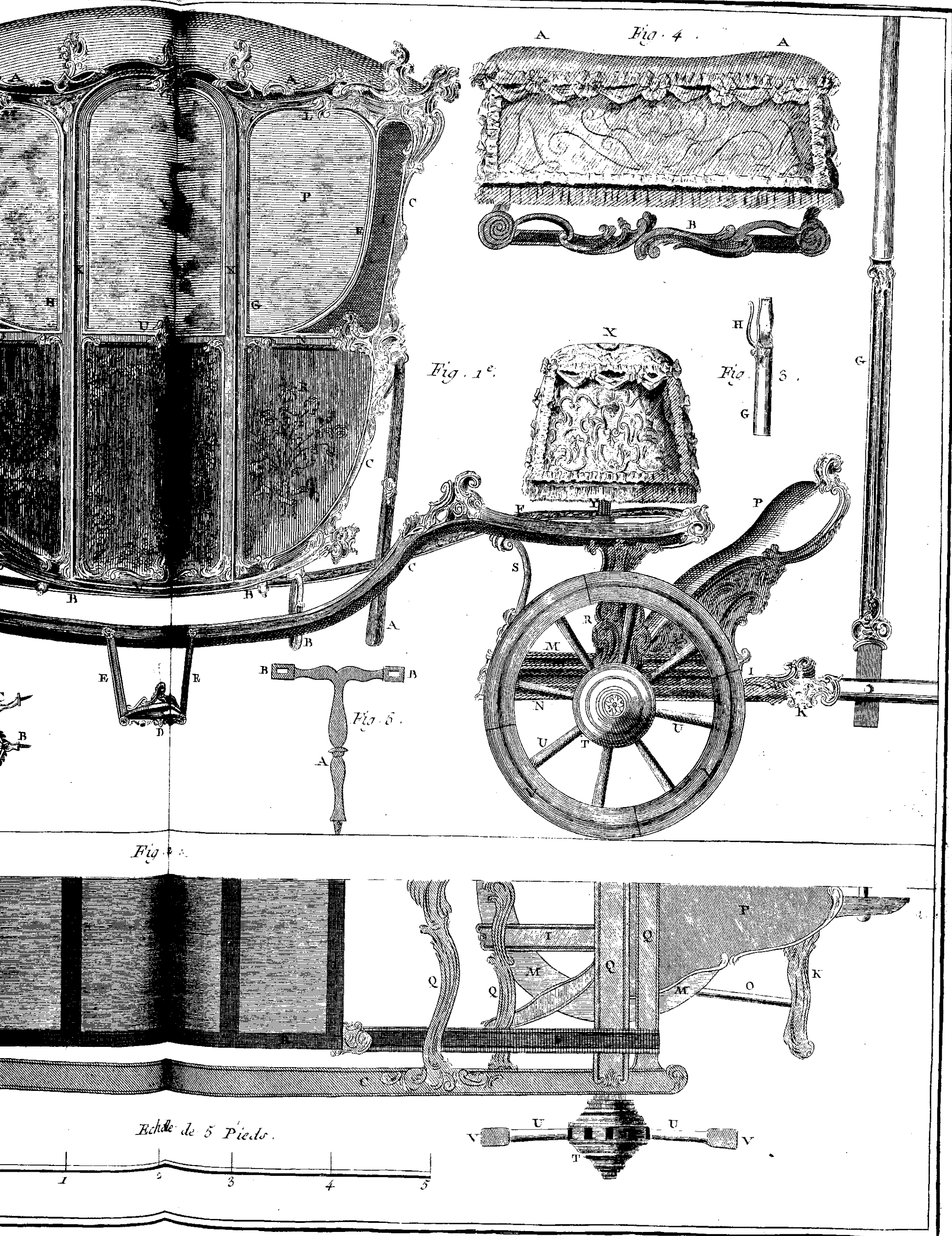
Carrossier, Berline ou vis-à-vis à deux Fonds.
