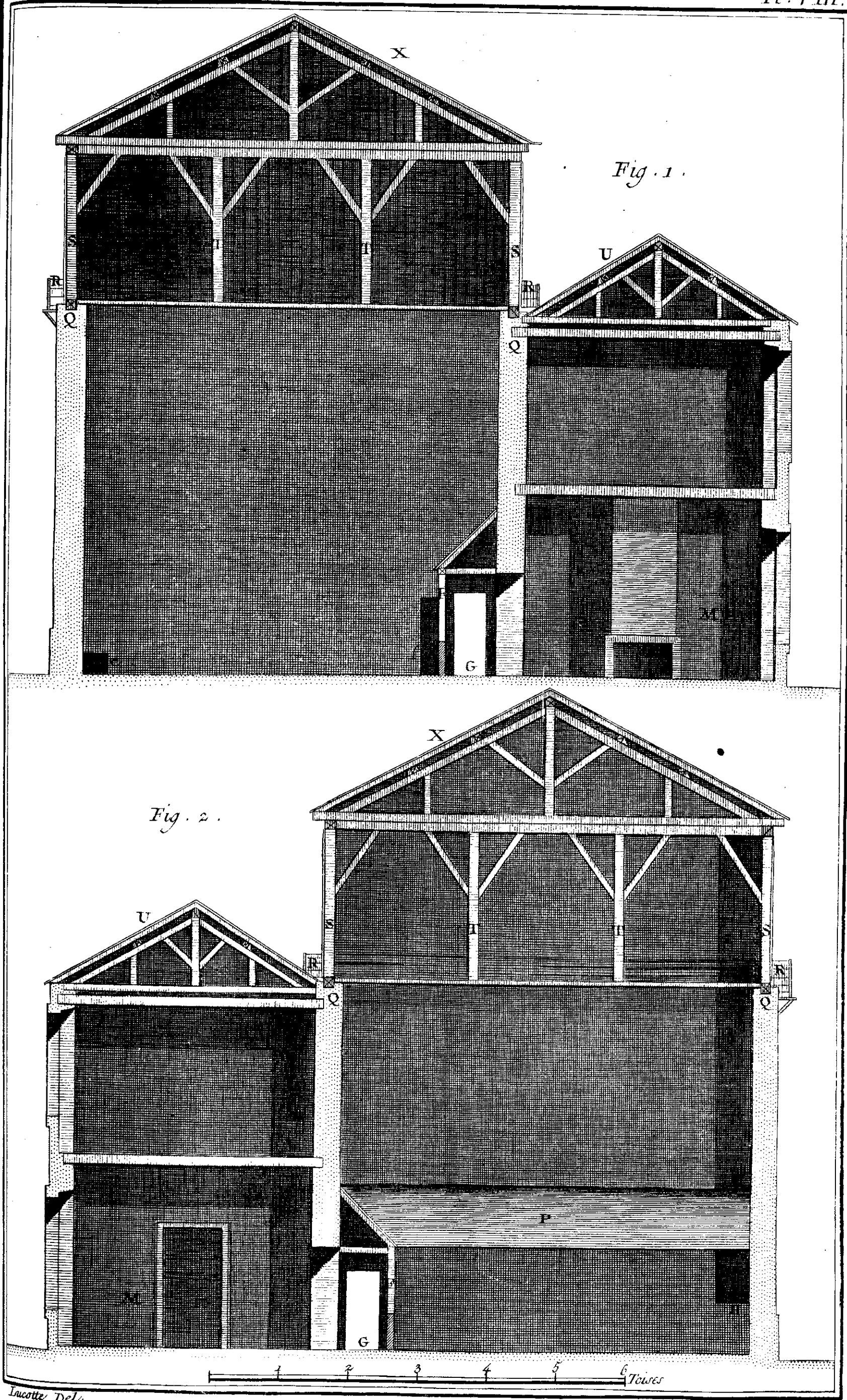
Paulmerie, coupes du Jeu de Paulme quarré.
