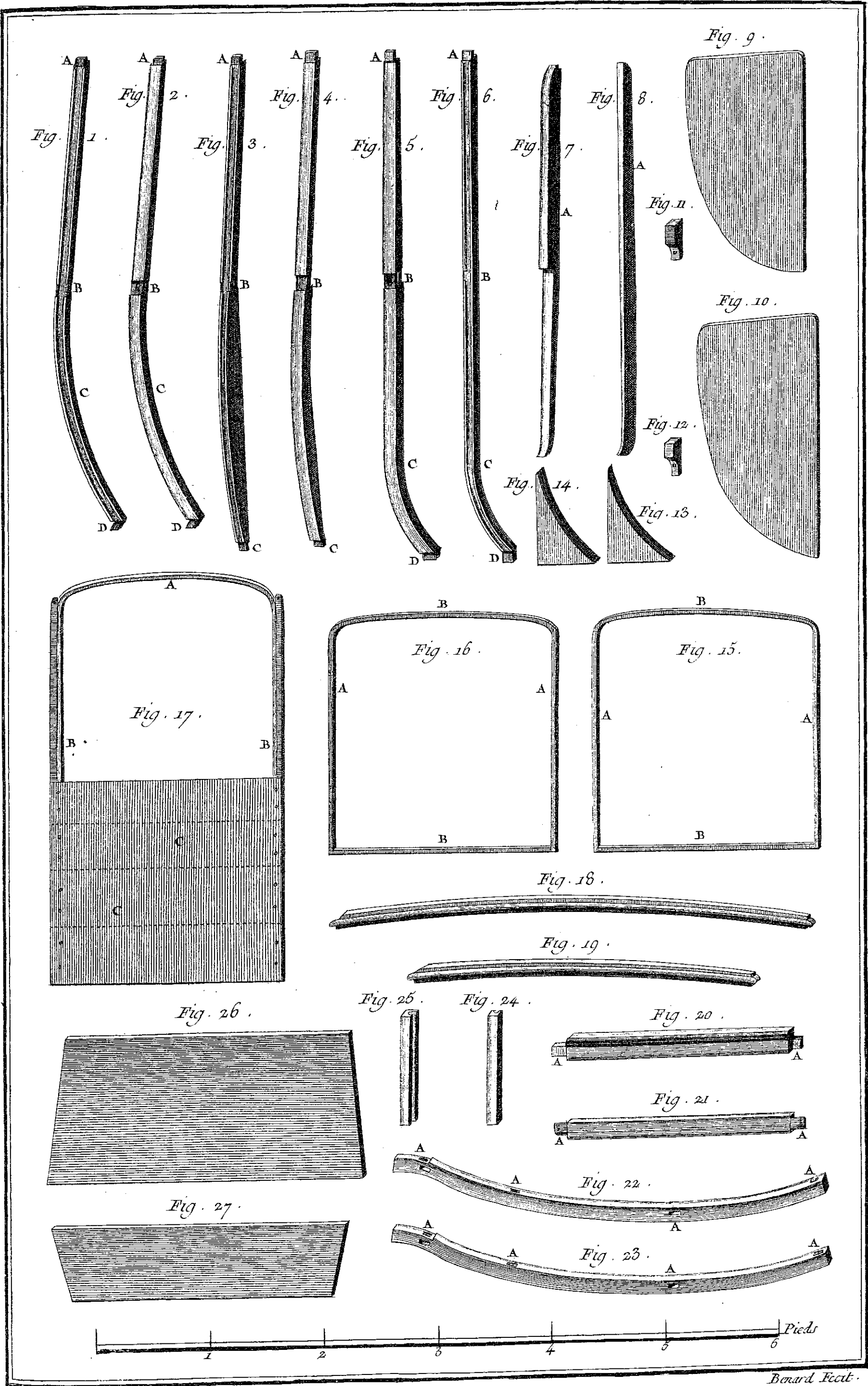
Menuisier en Voitures, Diligence à l'Anglaise, Détails.
