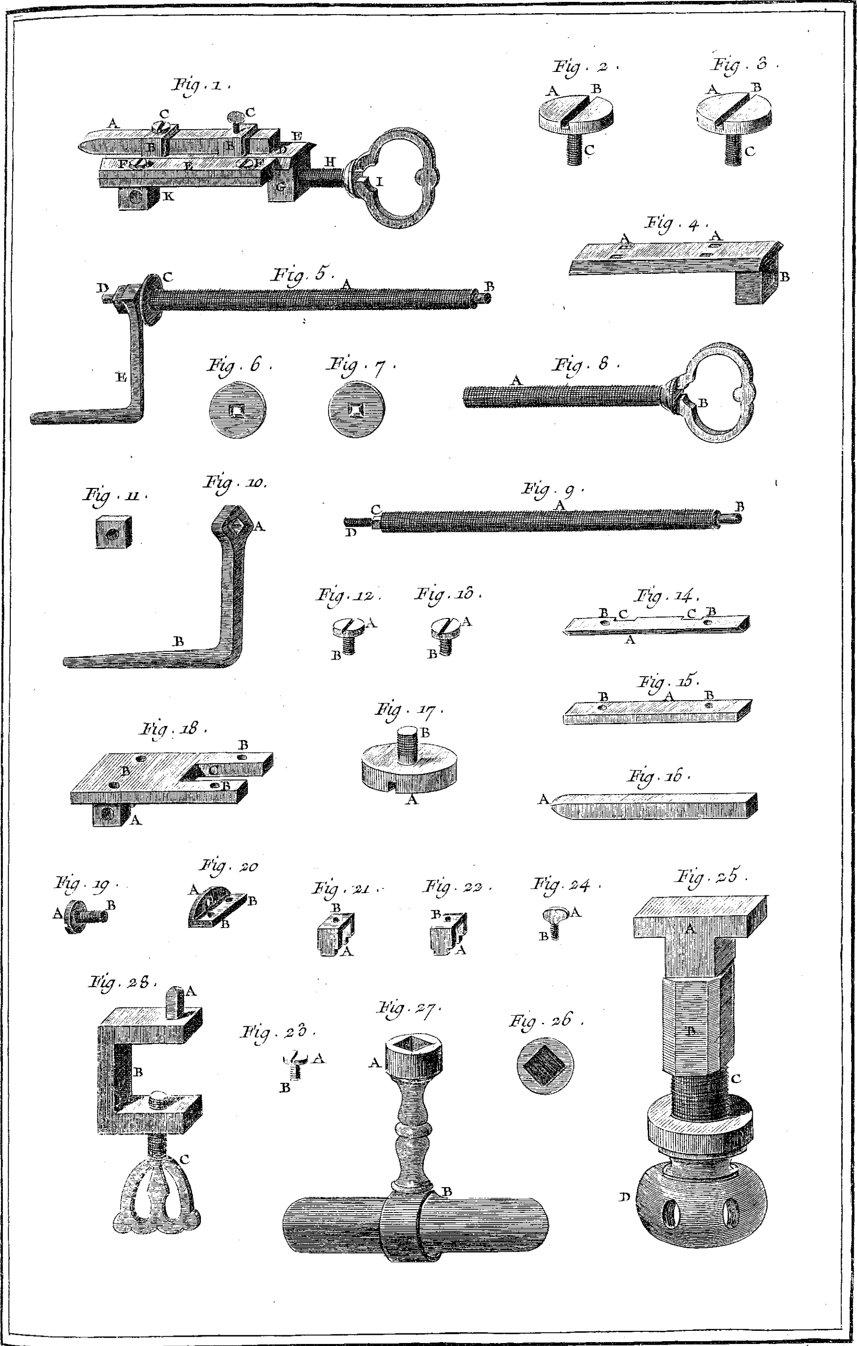
Tourneur, Tour à Figure, Détails du Support à pivot.
