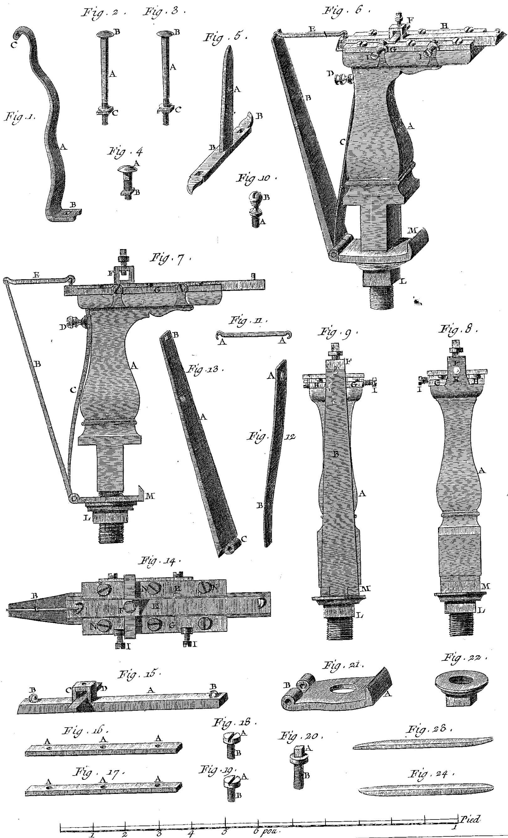
Tourneur, Tour à Figure, Support à Coulisse et ses Détails.
