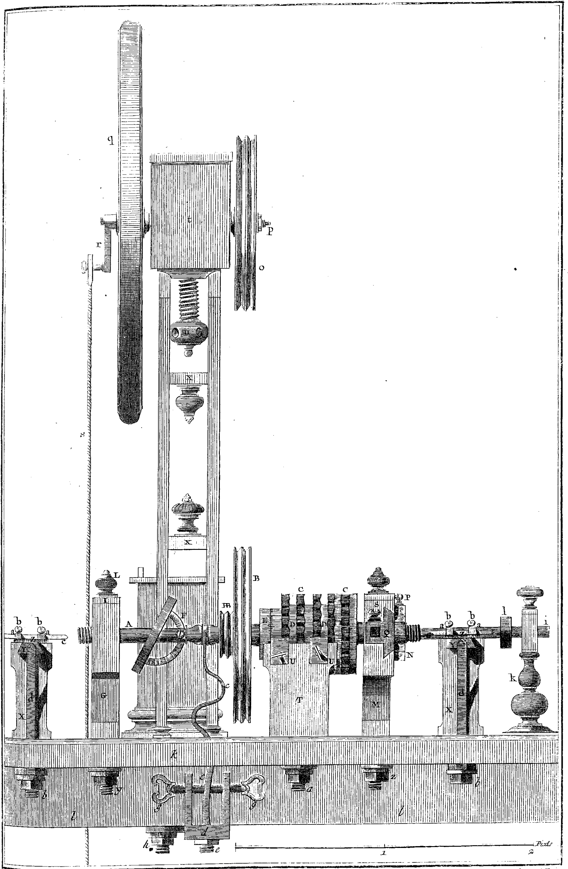
Tourneur, Tour à Guillochis avec Outils mobiles.
