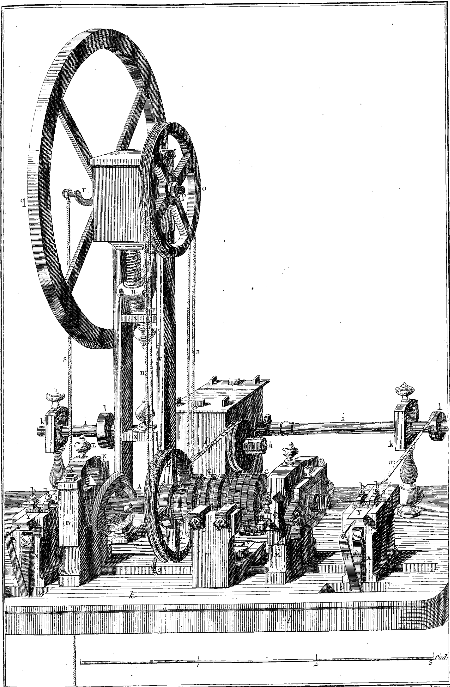
Tourneur, Tour à Rouë à Guillochis et Outils mobiles.
