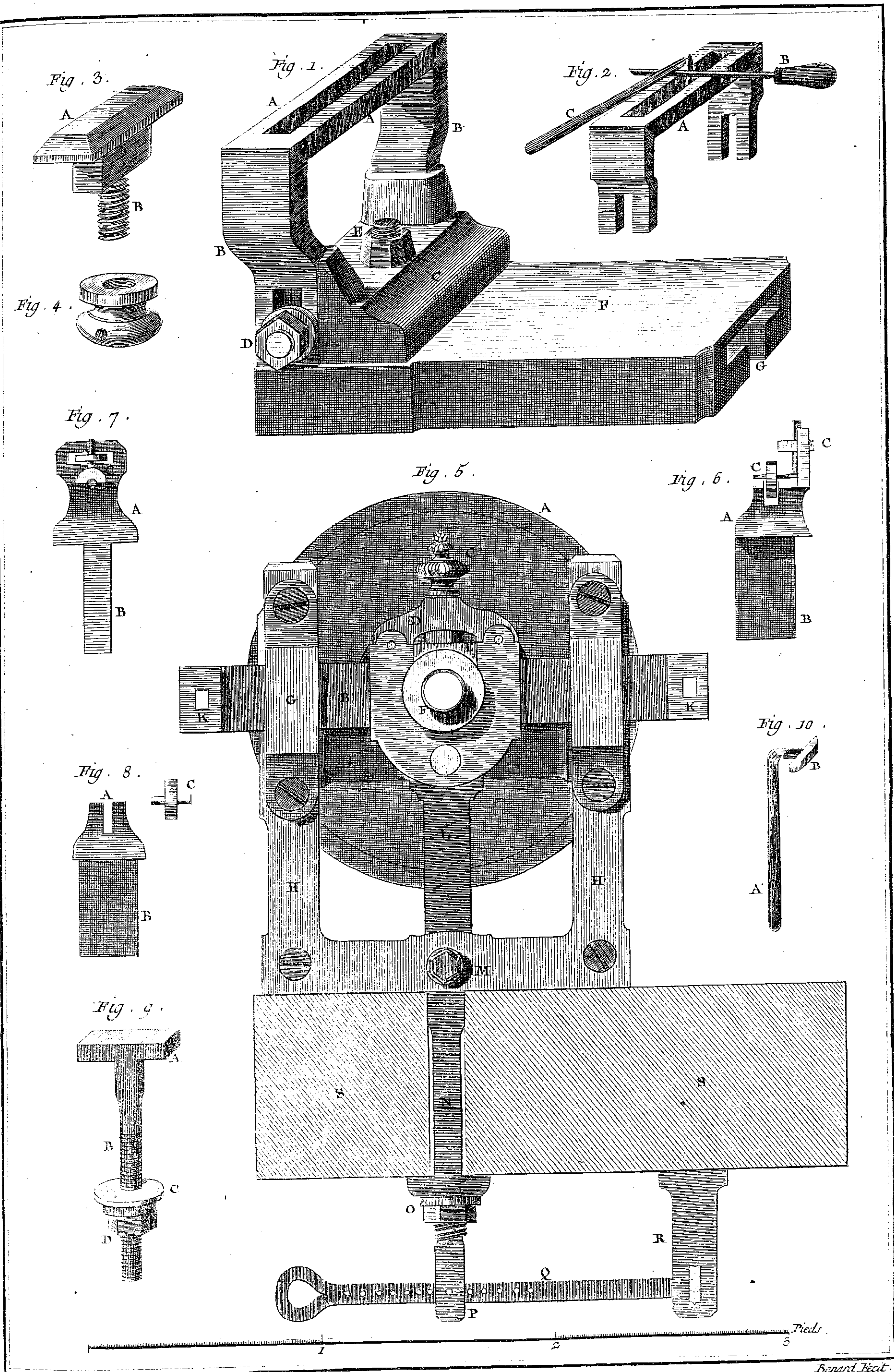
Tourneur, détails du Tour à Guillocher à Roue 2.
