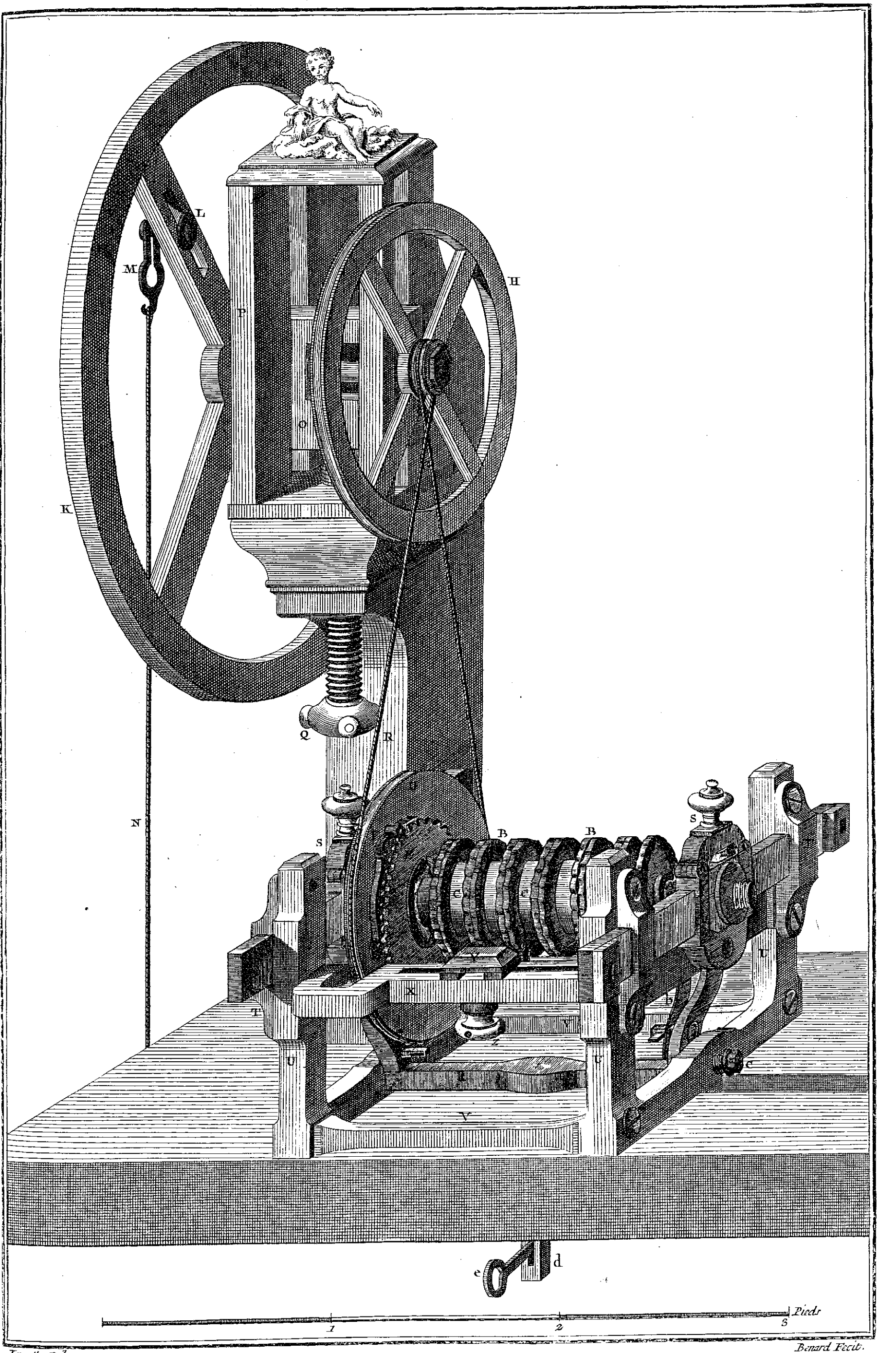
Tourneur, Tour à Guillocher à Roüe.
