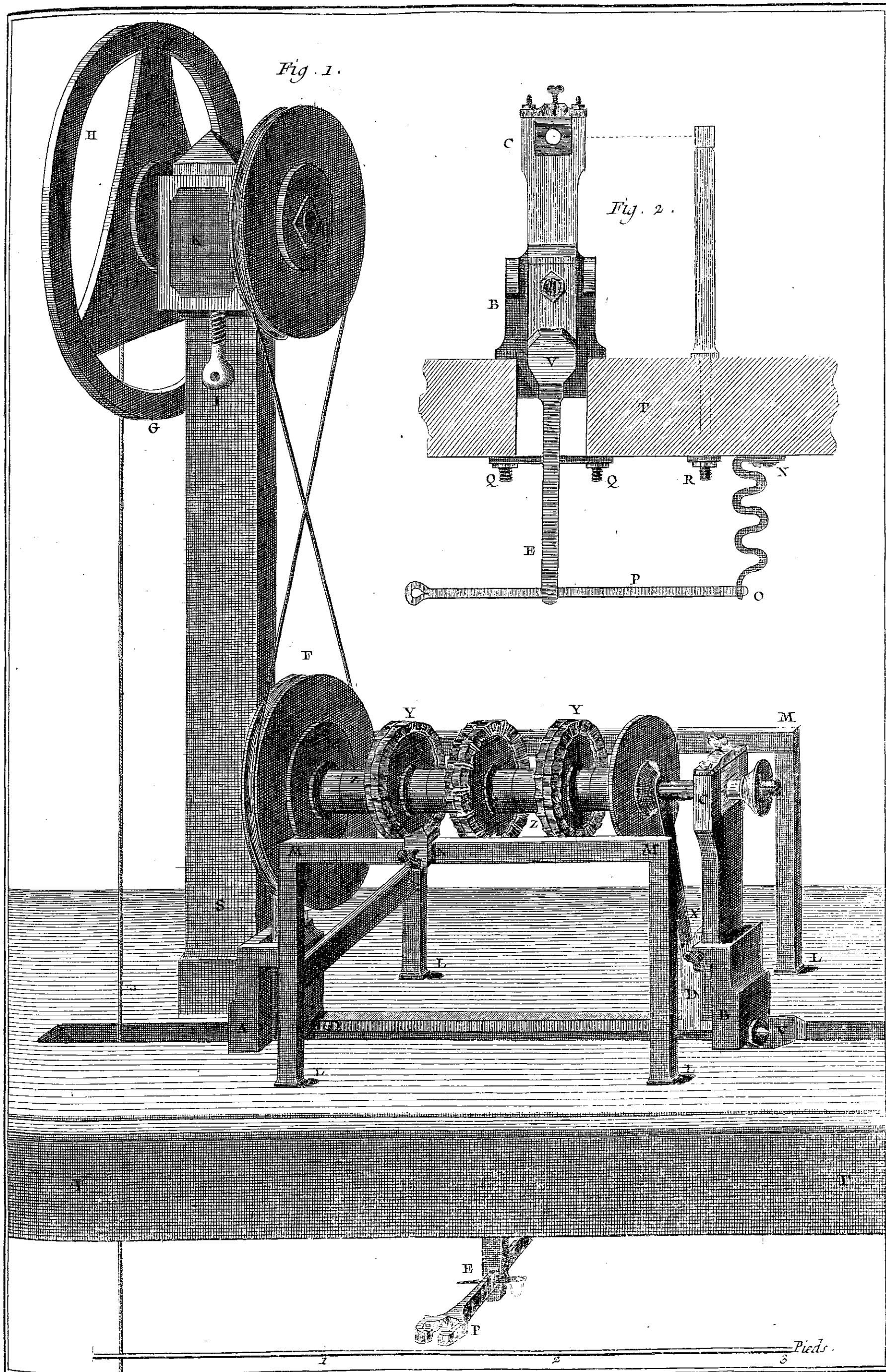
Tourneur, Tour à Guillocher à Rouë.
