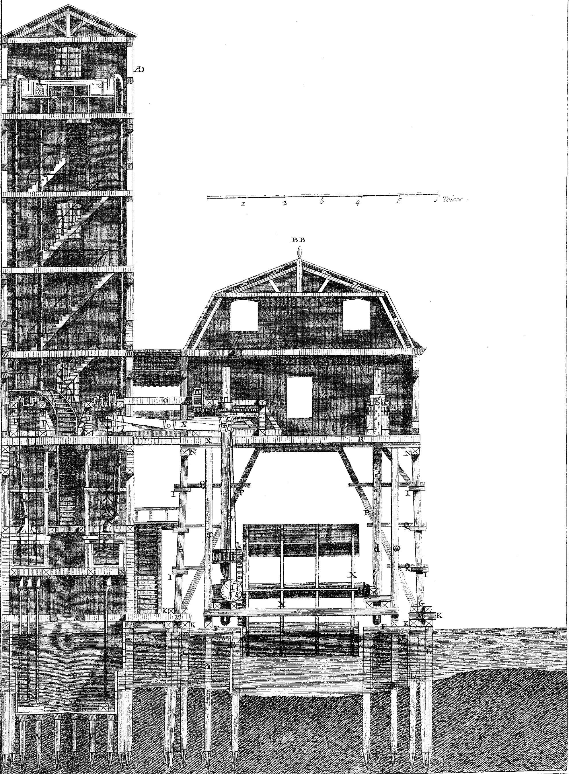
Charpente: Pompe du Pont Notre-Dame.
