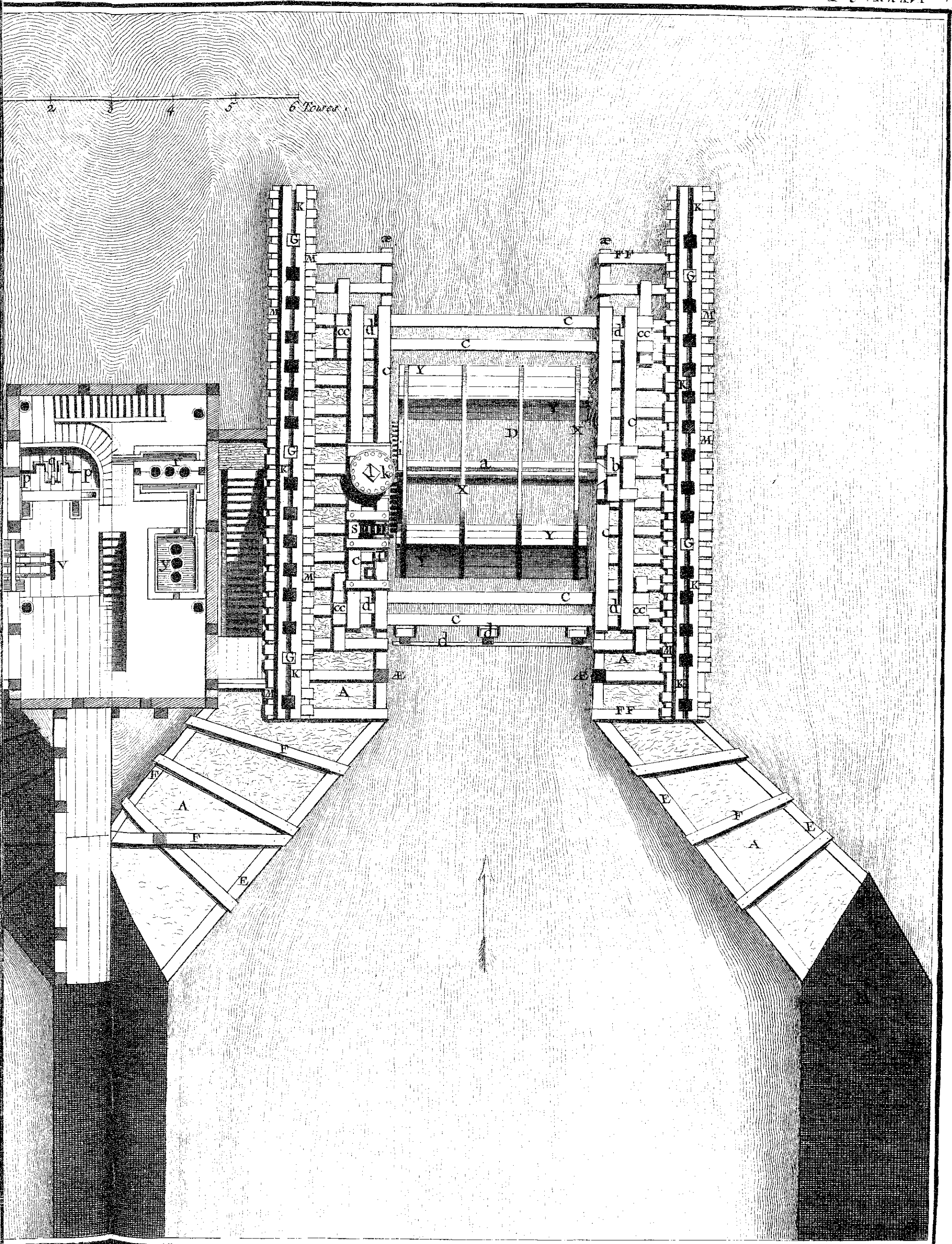
Charpente, Pompe du Pont Notre Dame
