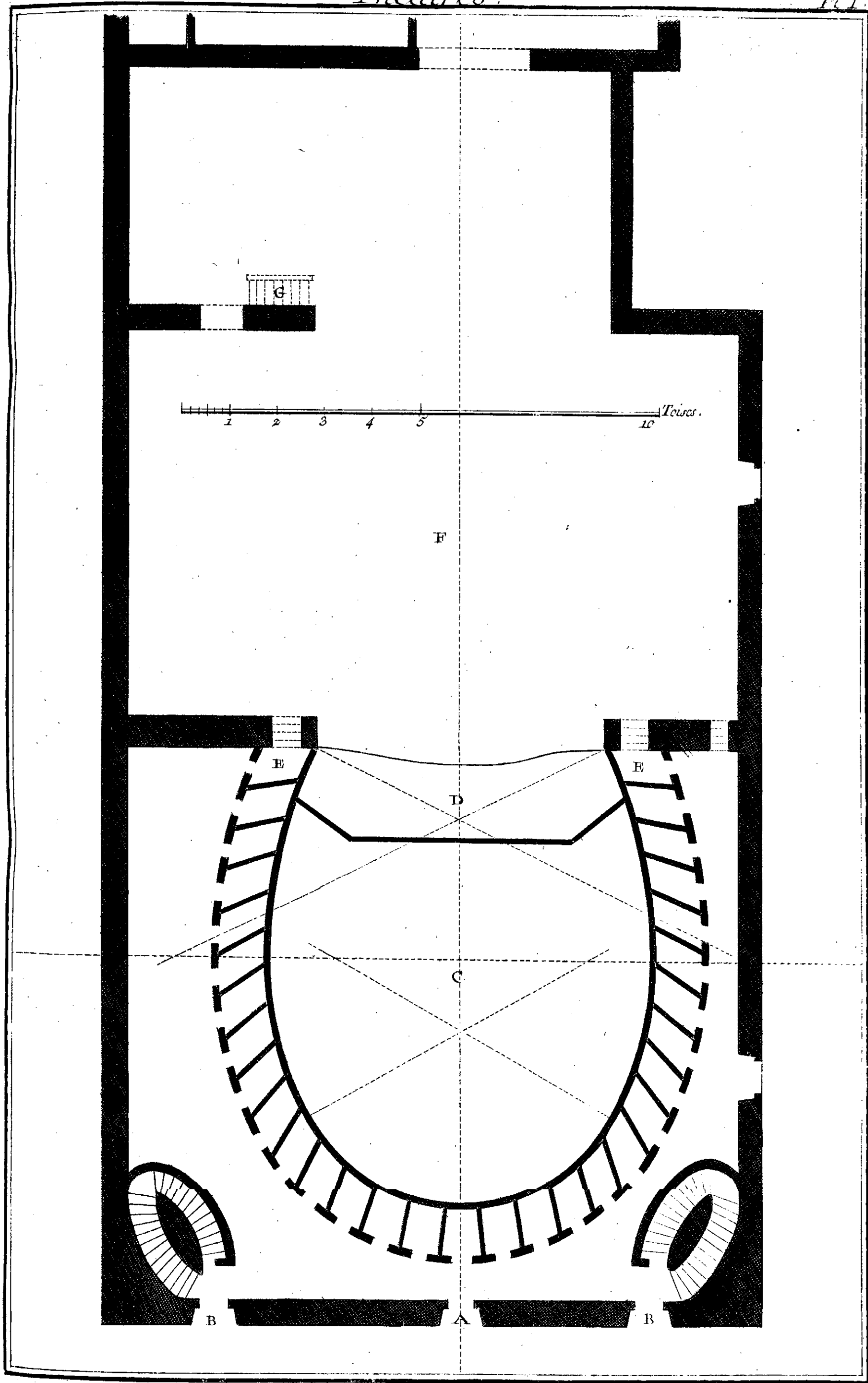
Salles de Spectacles. Plan du Theatre d'Argentine à Rome.
