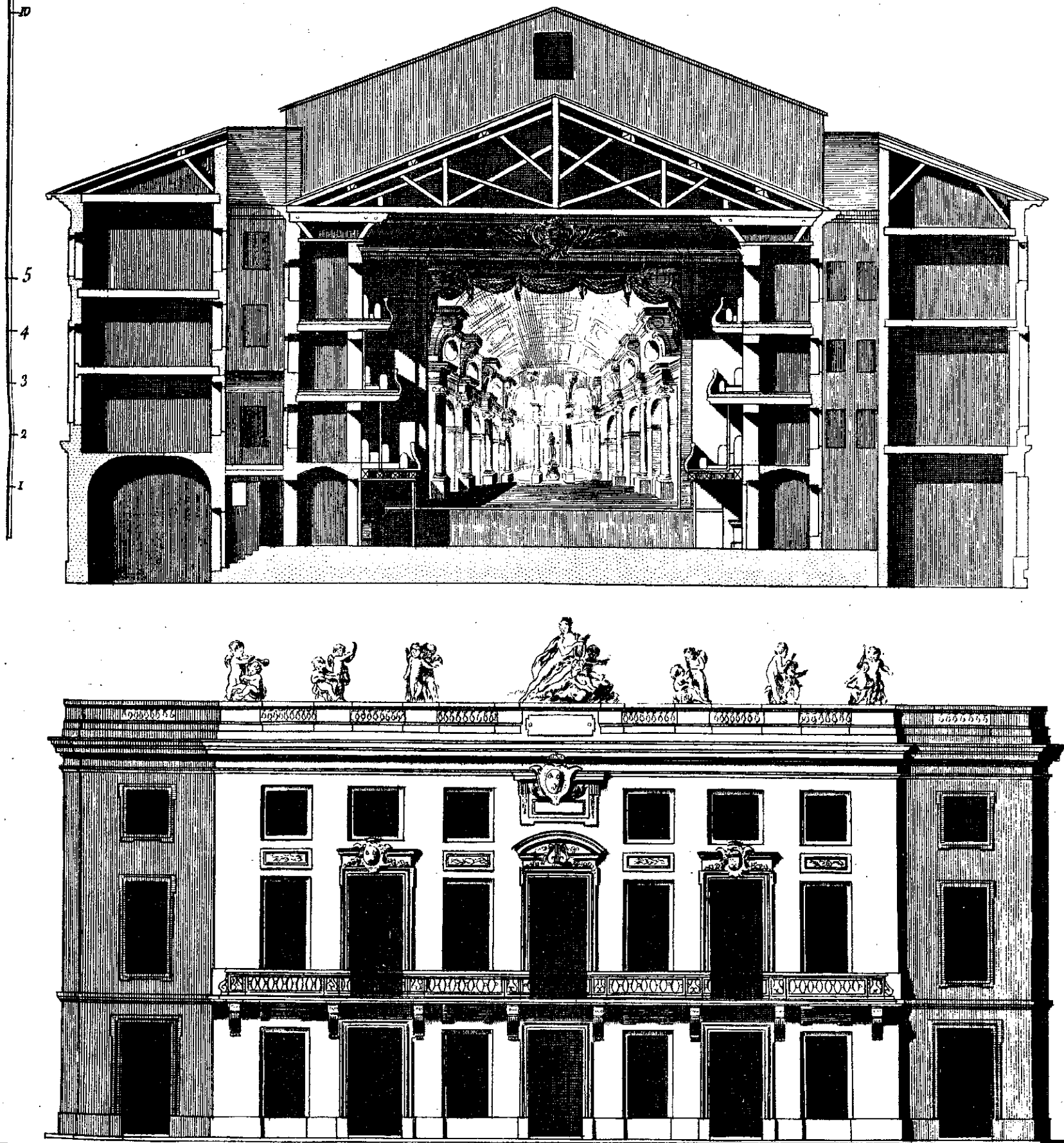
Salles de Spectacles Coupes et Élévations de la Salle de Comédie de Lyon.
