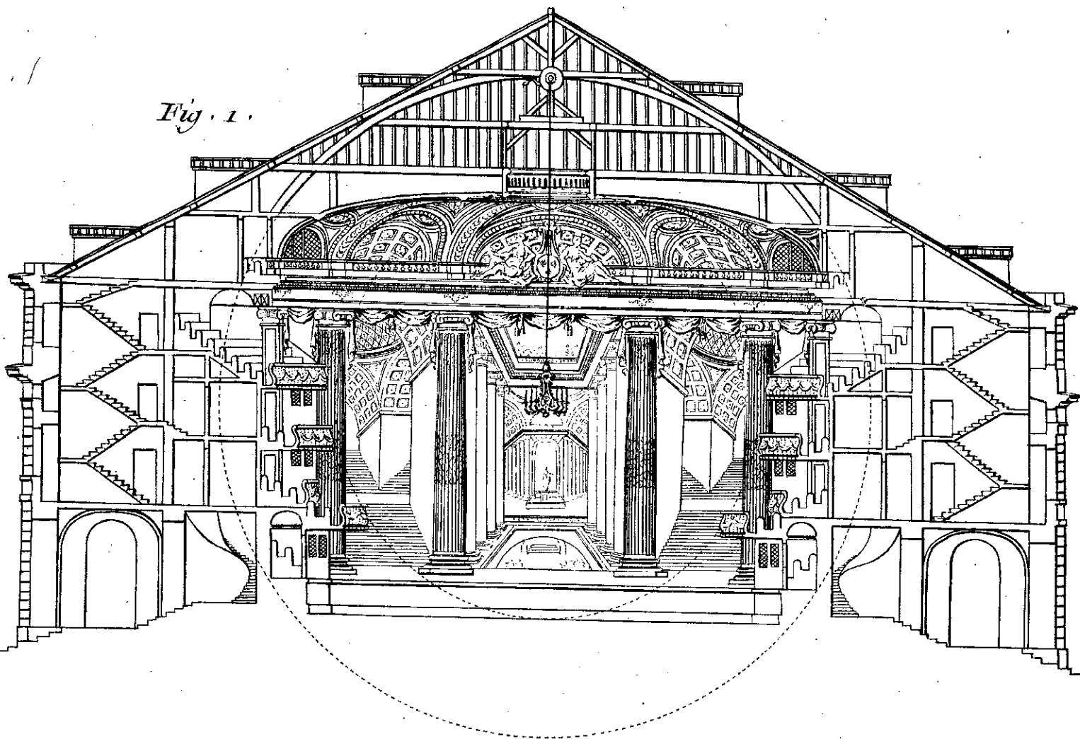
Coupe en face du Théâtre.
