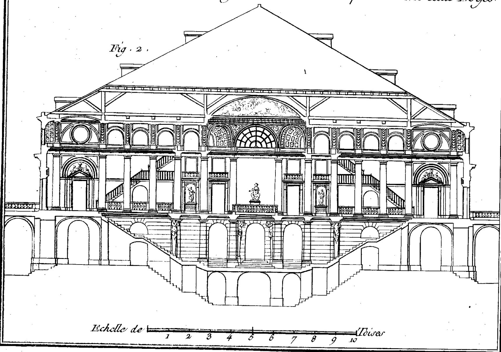
Coupe du foyer public et des grands Escaliers qui montent aux Loges.
