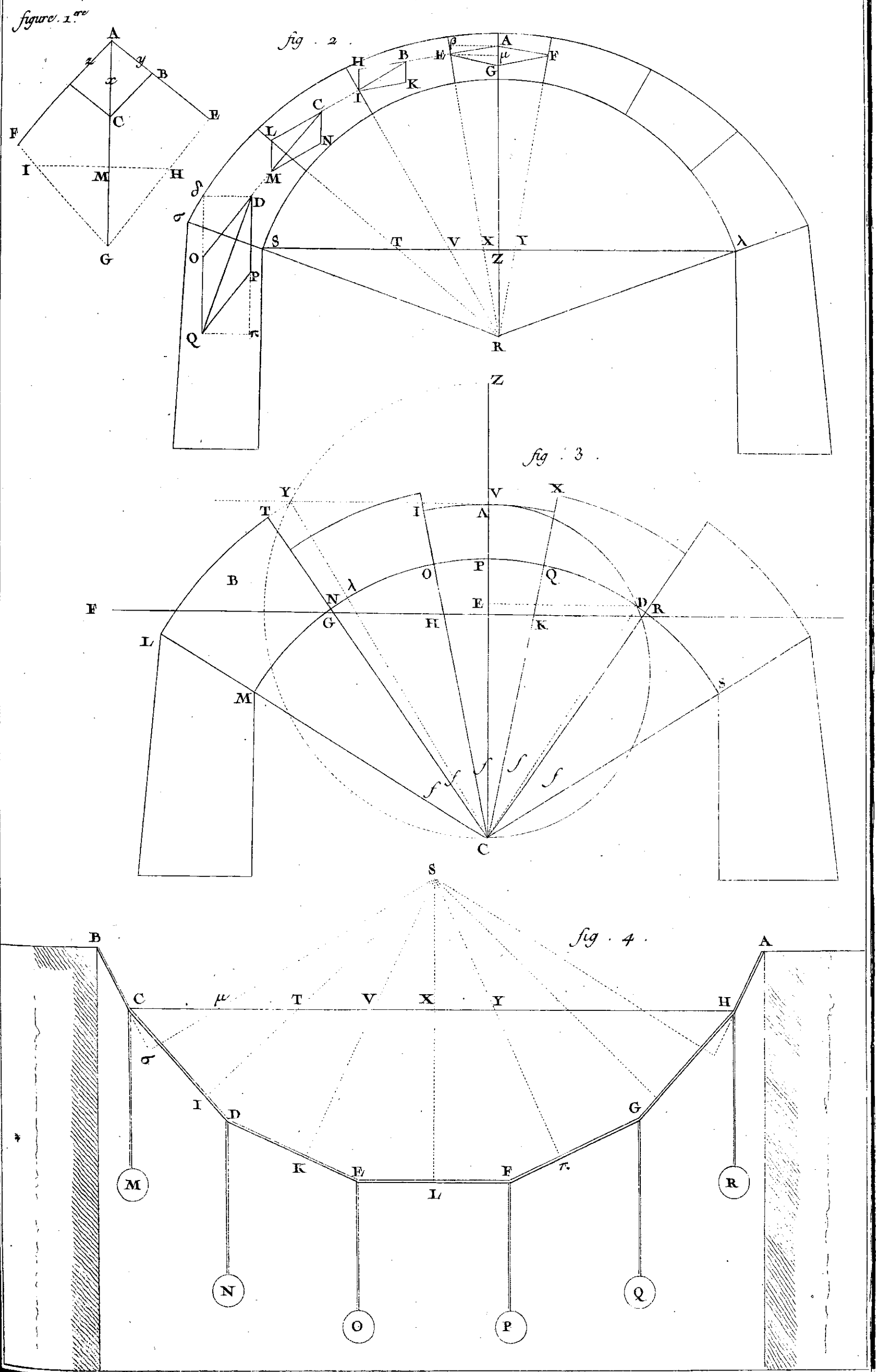
Architecture, Coupe des Pierres.
