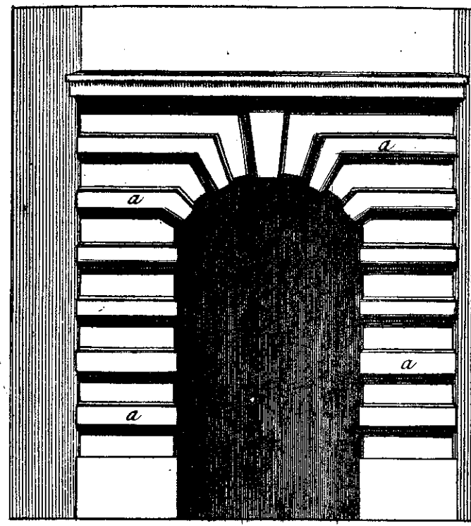
Porte Dorique.
