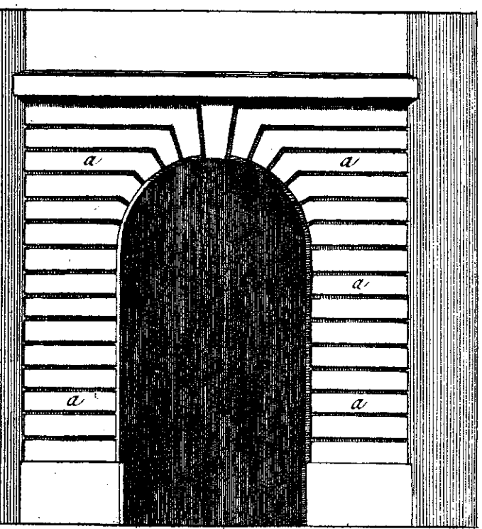
Porte Ionique.
