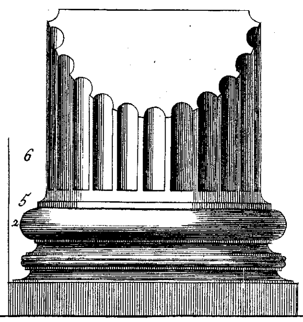
Base Ionique.
