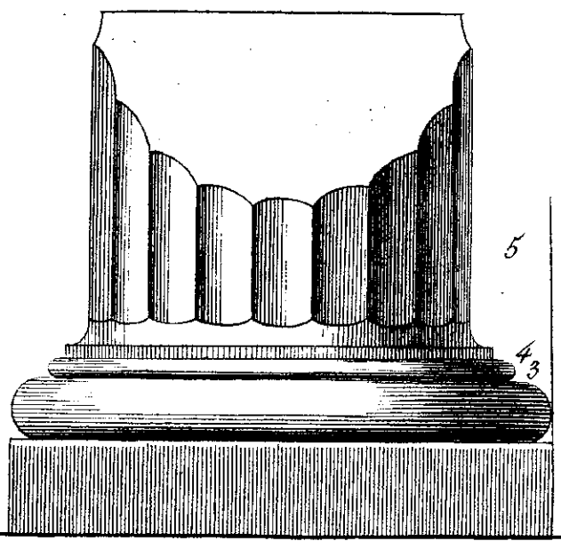
Base Dorique.
