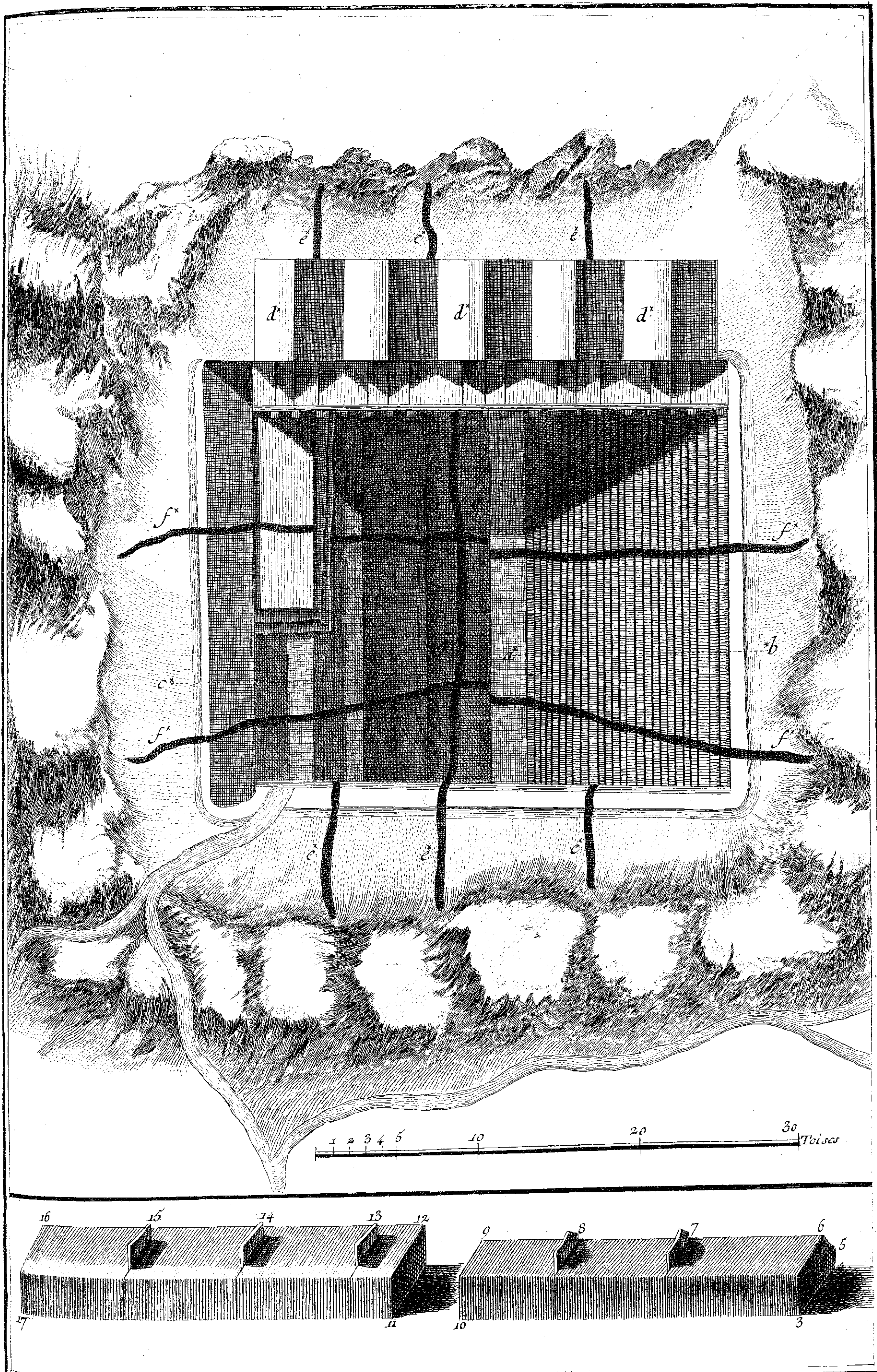
Minéralogie, Plan d'une carrière d'Ardoise près d'Angers
