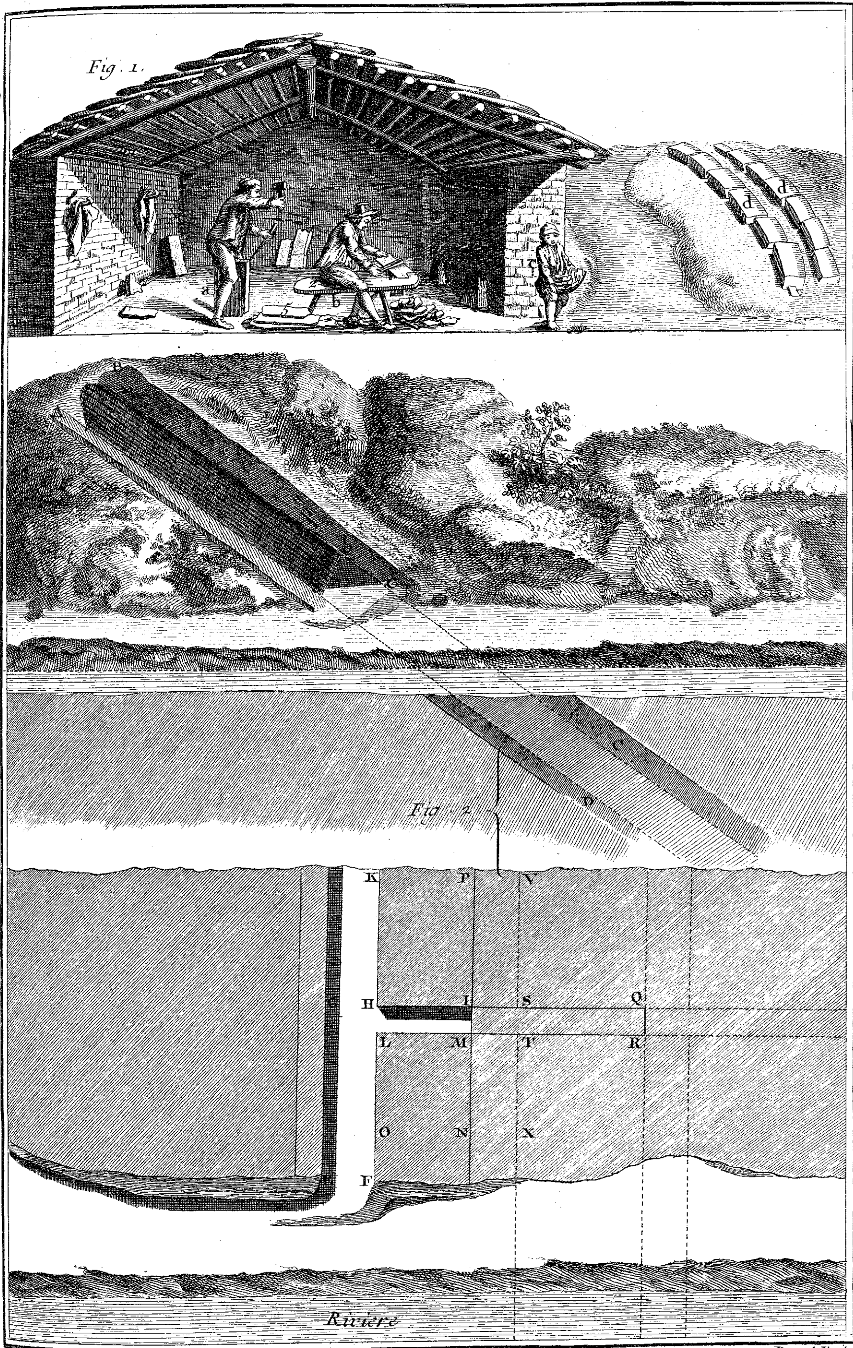
Minéralogie, Ardoiserie de la Meuse. Atelier pour le travail des ardoises et Plan et Profil d'un Banc d'Ardoise moins épais que celui de Rimogne.
