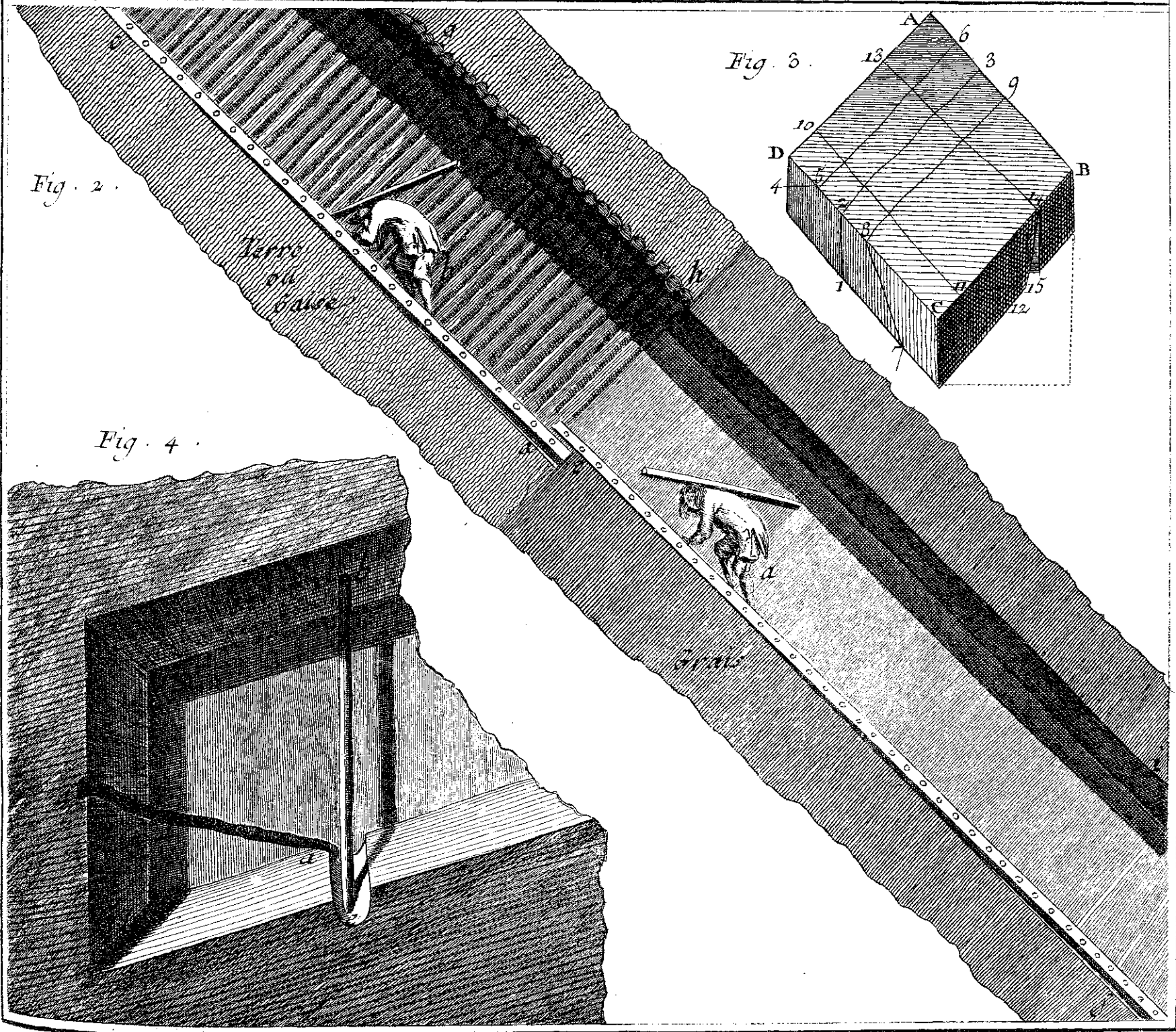
Minéralogie, Ardoiserie de la Meuse. Vue perspective d'une culée et de ses sept longueurs et coupe d'une gallerie inclinée.
