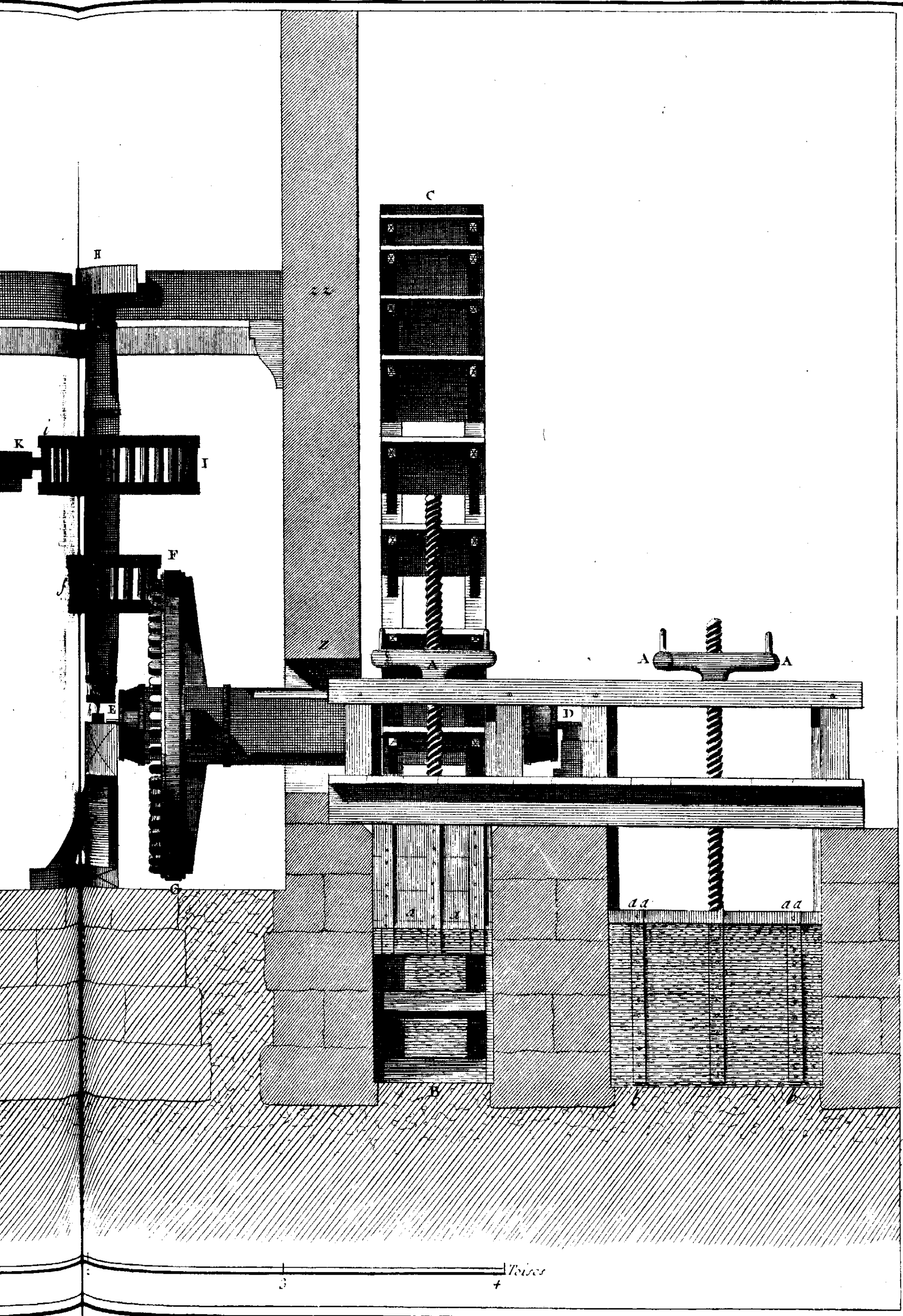
Poudre Canon. Élévation Longitudinale du Moulin à meules roulantes.
