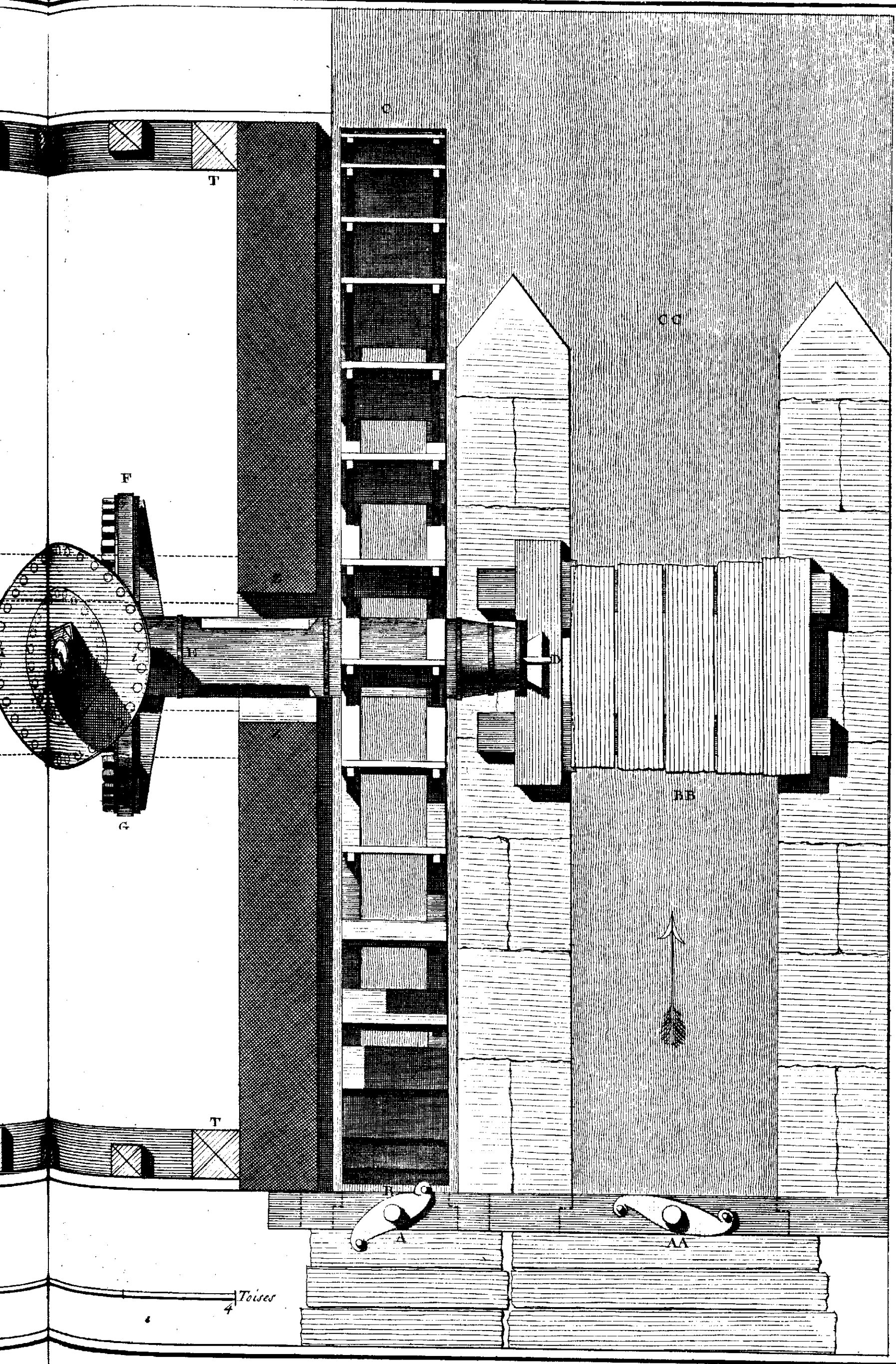
Moulin à Canon . Plan du Moulin à Meules roulantes .
