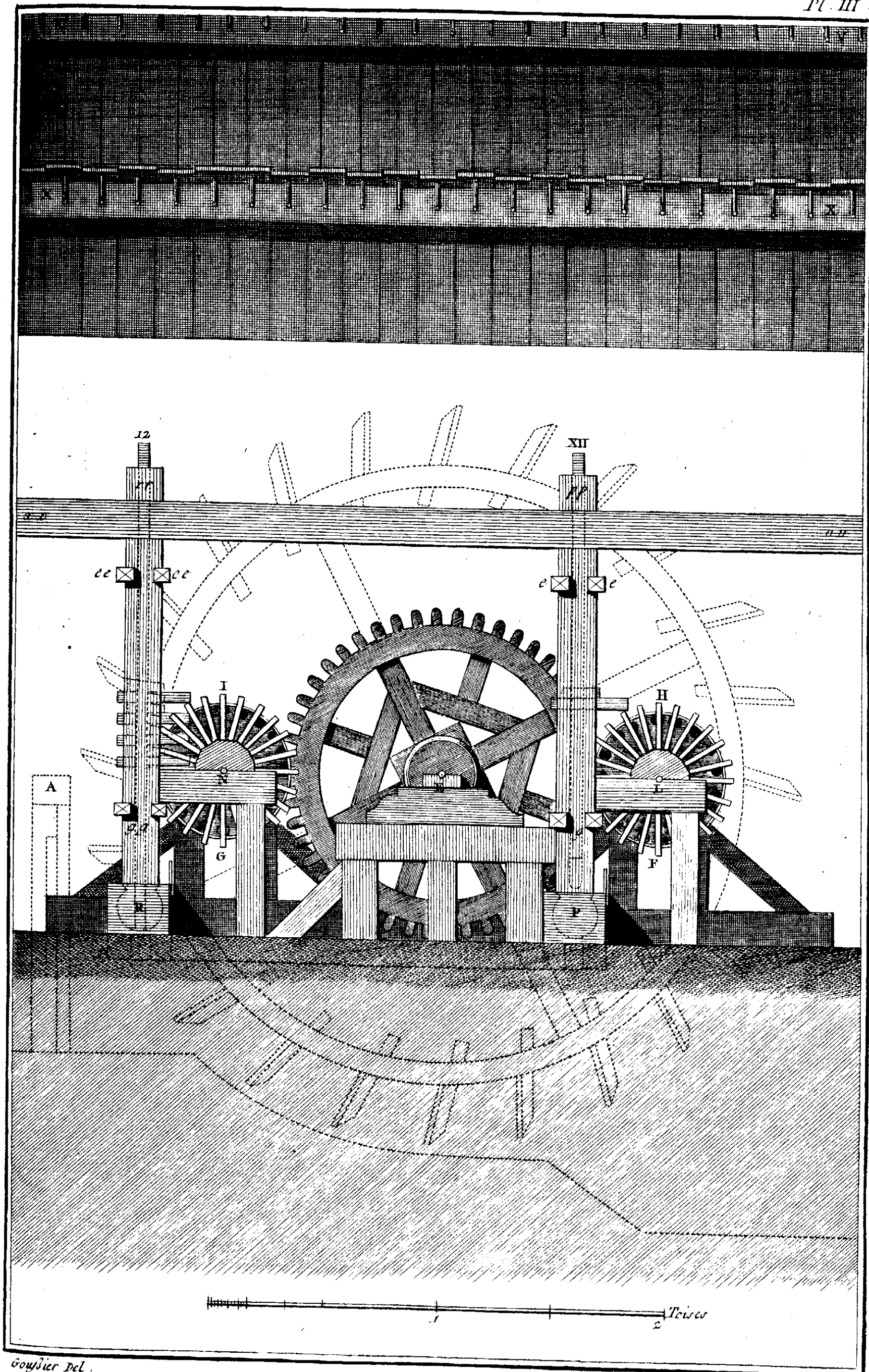
Minéralogie, Fabrique de la Poudre à Canon. Profil du Moulin à Pile.
