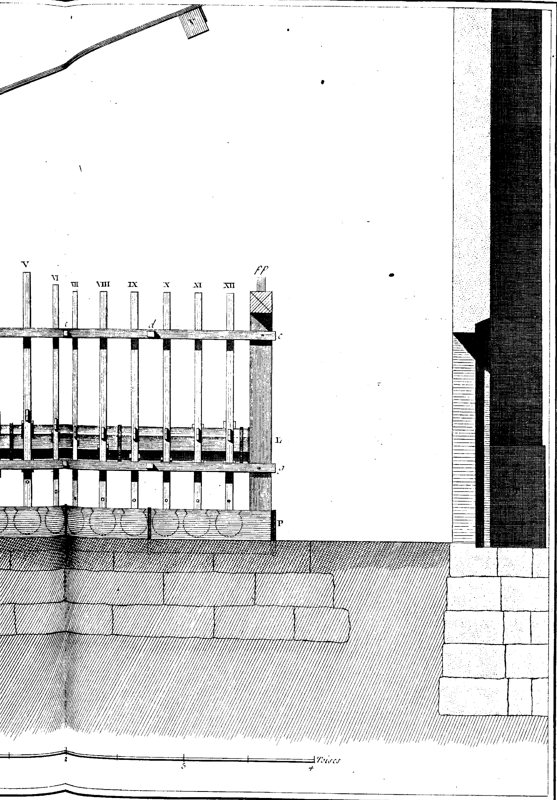
de la Poudre à Canon. Élévation du Moulin à Pylons.
