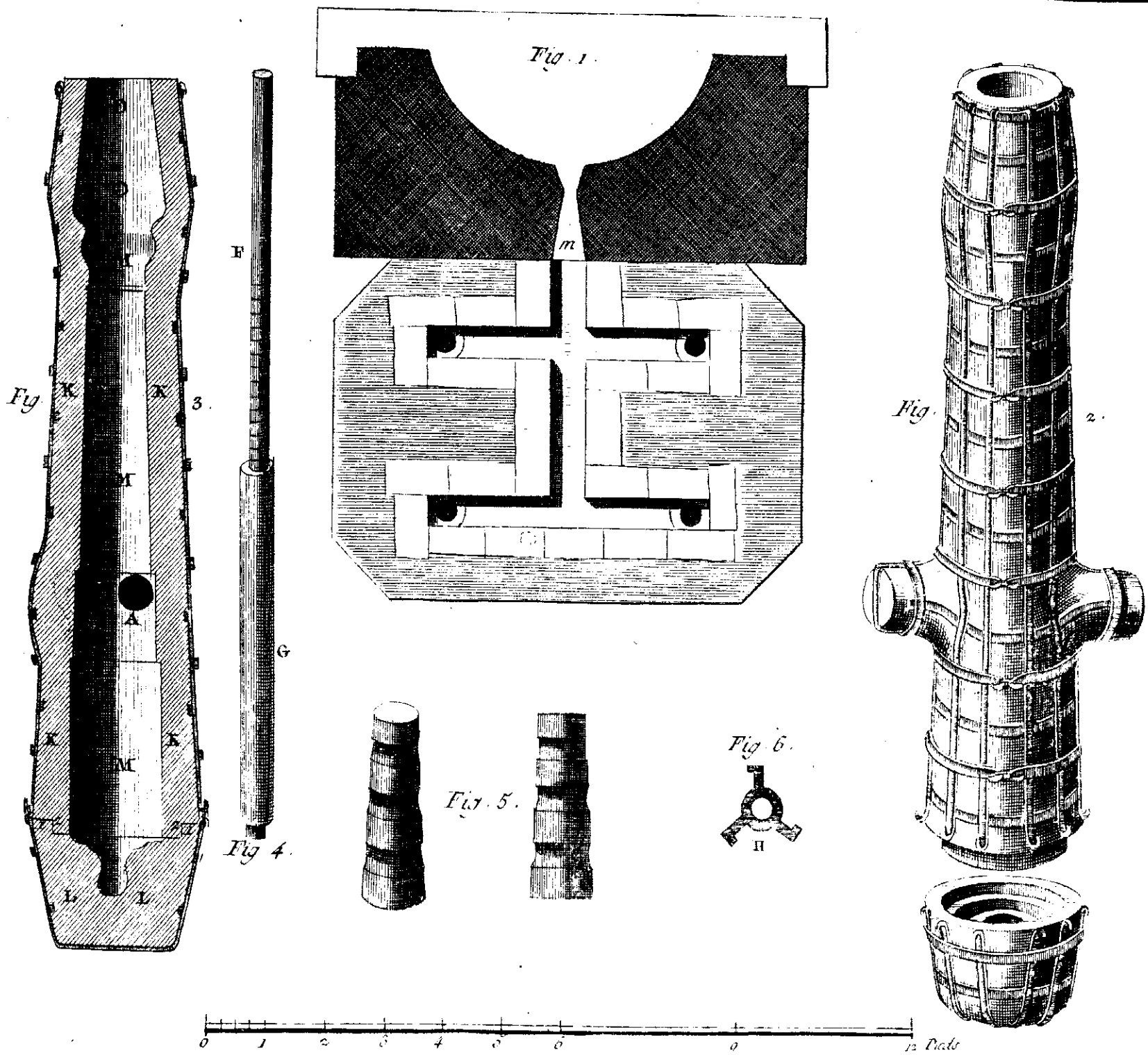
Fonte des Canons, l'opération de Secher les Moules, Plan de l'Atelier 3...
