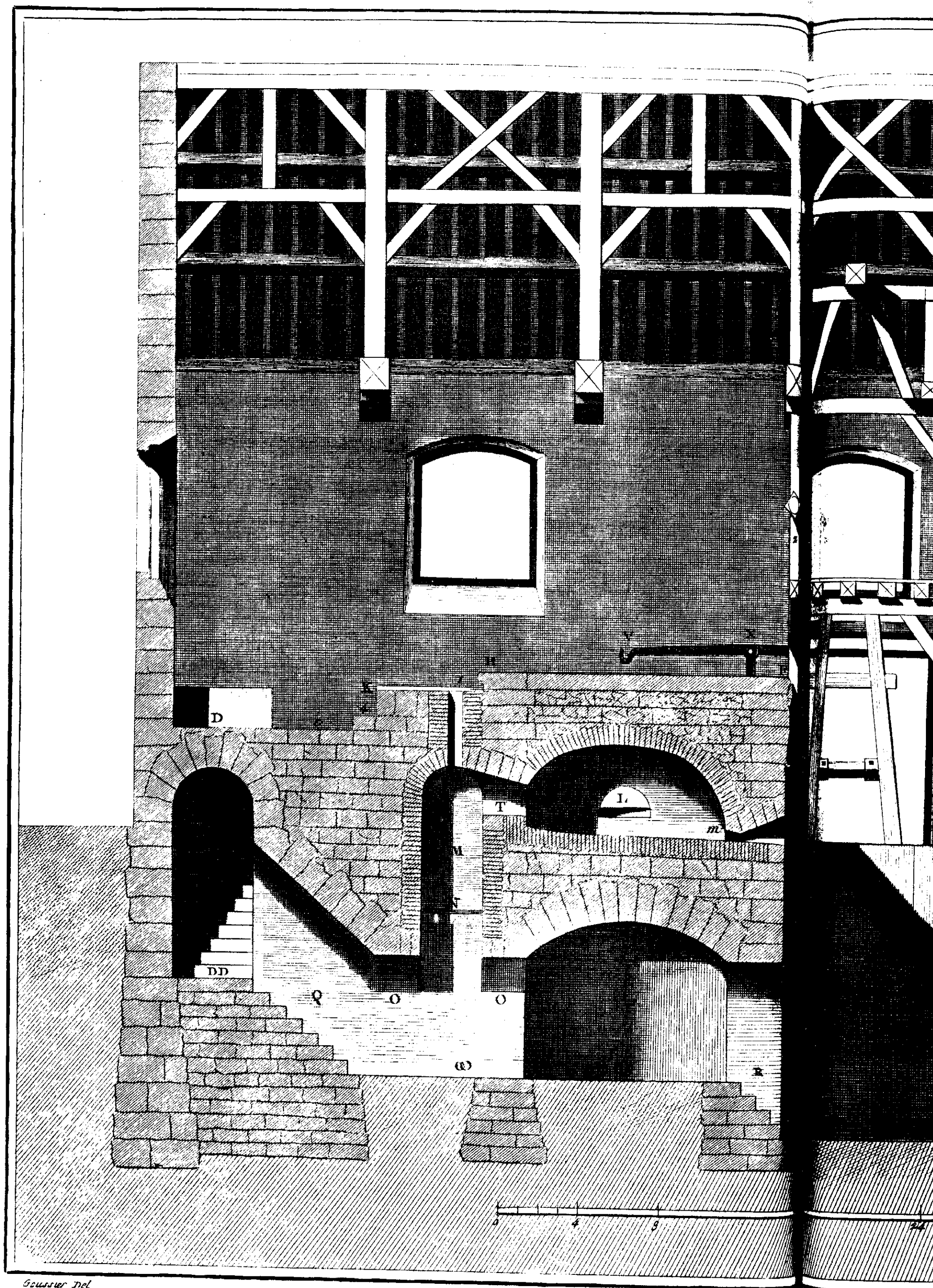
Fonderie des Canons, coupe Longitudinale du Fourneau pour la chauffe, ca
