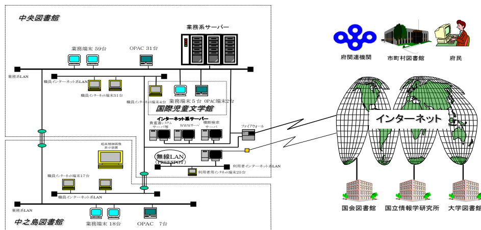
大阪府立図書館コンピュータシステムハードウェア構成図
