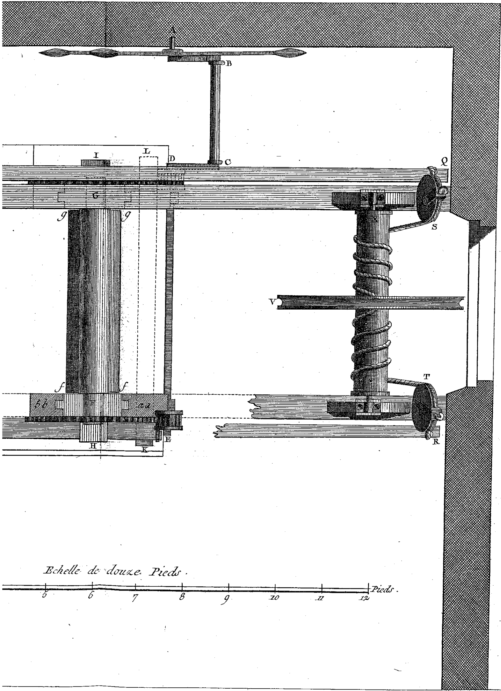
De la Machine servant à Cilindrer les Étoffes.
