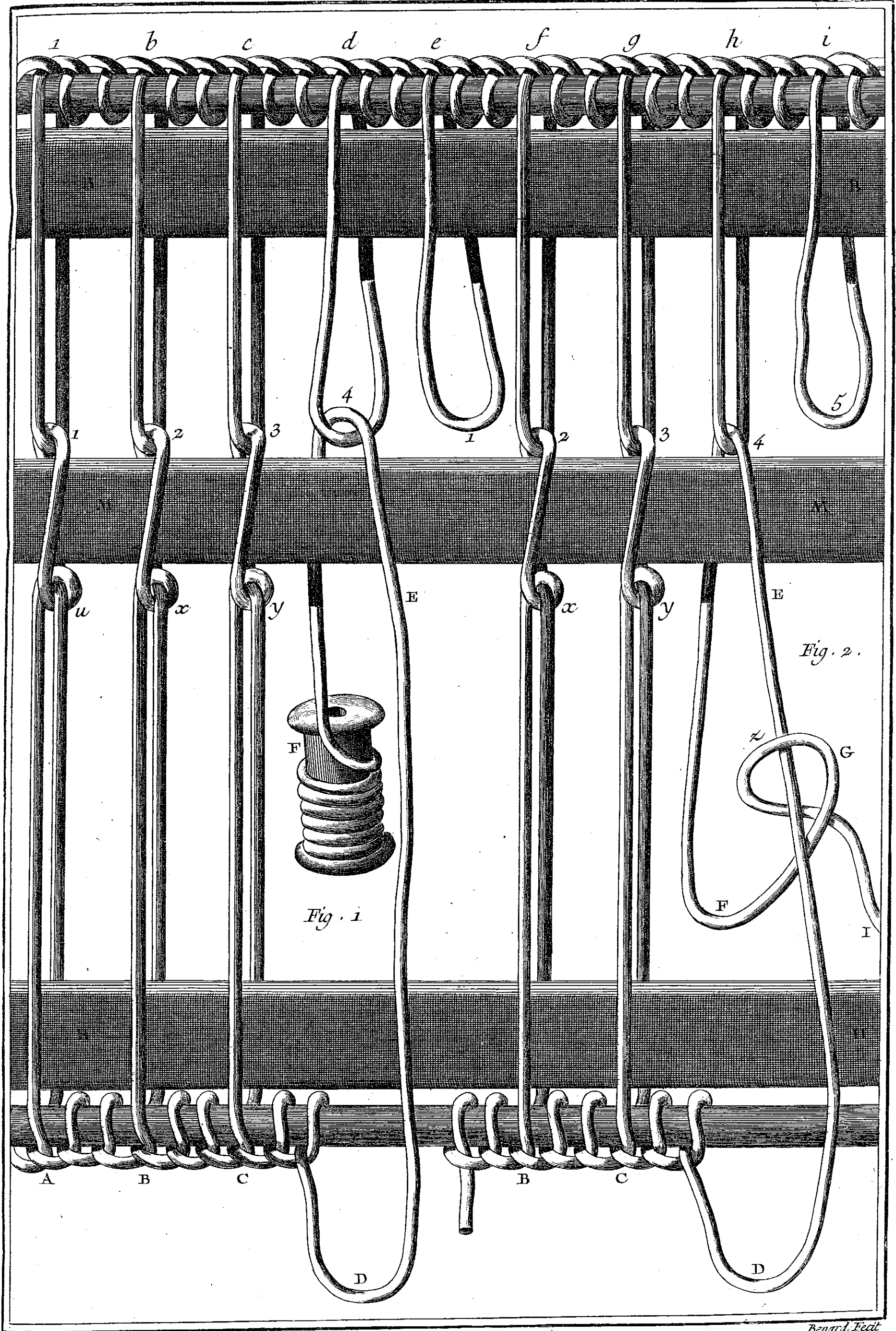
Soierie, Lisses à Nœuds. premier et second temps de la formation de la maille.
