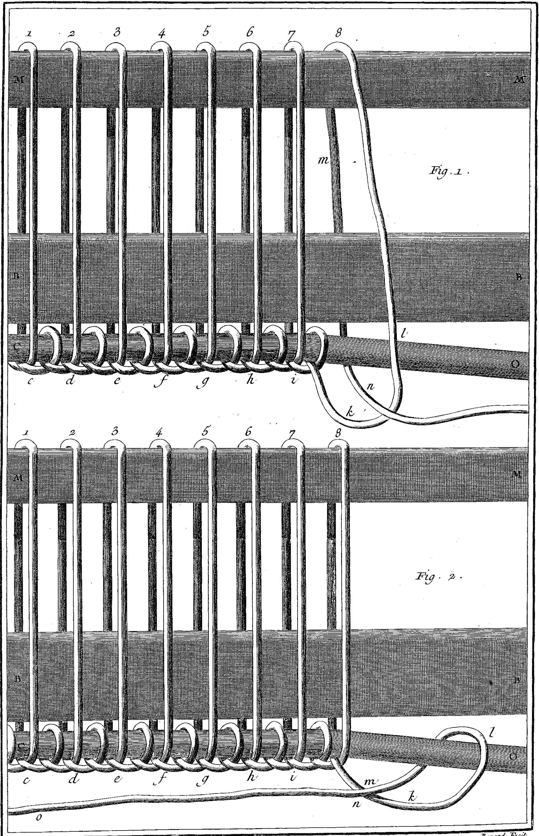
Soierie, Formation du Bas des Lisses et Maniere de Natter.
