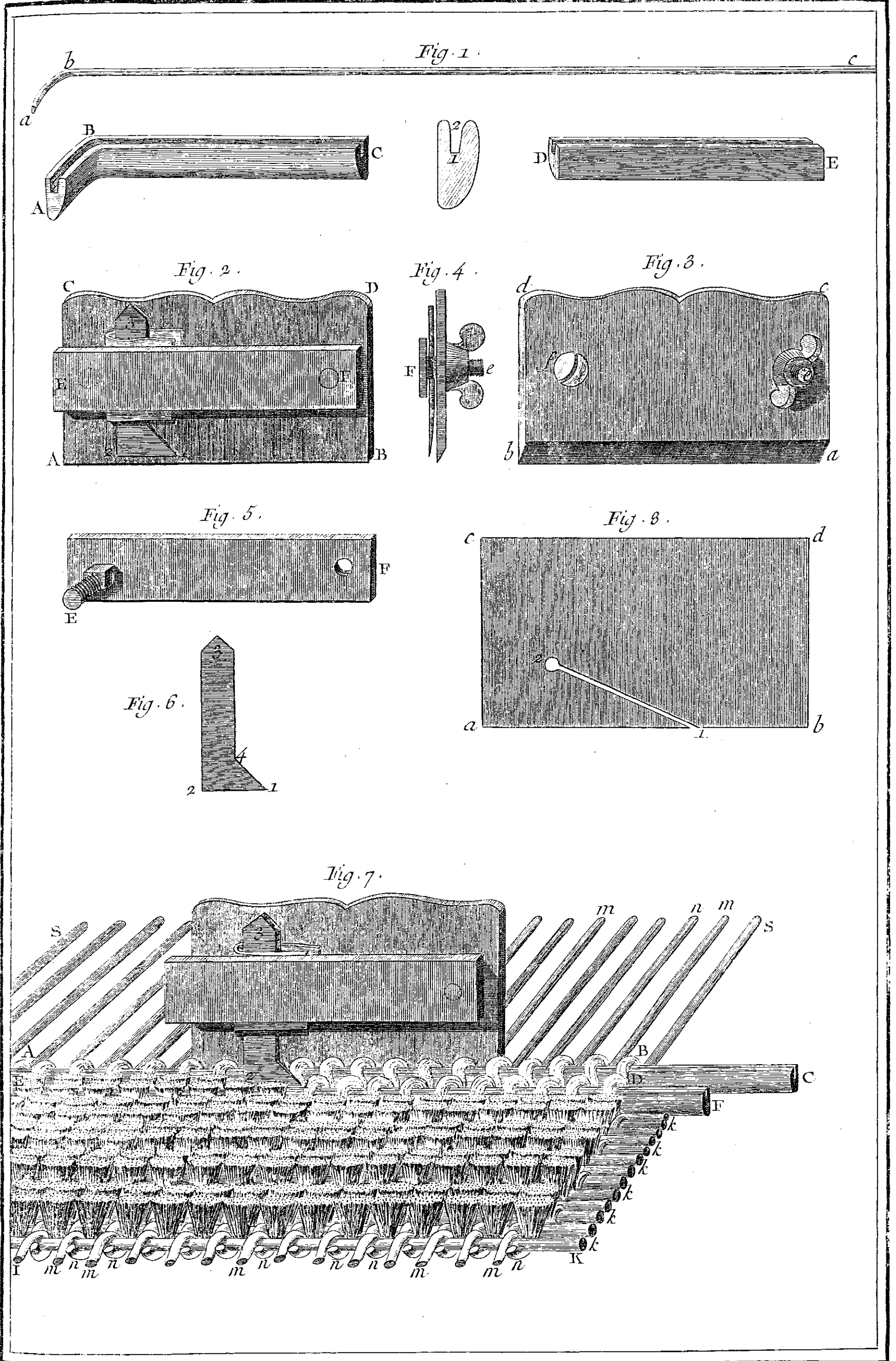
Soierie, Vélours Coupé. Fers de Coupé, Rabot, m m m Taillerolle: Usage du Rabot et Vélours Coupé vu au Microscope et en perspective.
